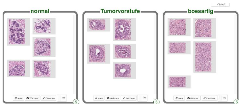
Abb. 2 Trainingsansicht MLforKids 10
