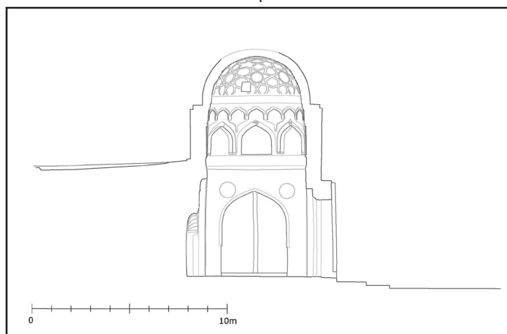
تصویر b4. مقطع شمالی - جنوبی مسجد جامع قرهه. (اسکن: یاسمین بدر. ترسیم: یولیا مولر).
