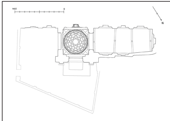
تصویر ۳. پلان مسجد جامع قرهه (اسکن: یاسمین بدر. ترسیم: یولیا مولر).
