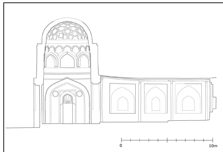
تصویر a4. مقطع شرقی - غربی مسجد جامع قرهه (اسکن: یاسمین بدر. ترسیم: یولیا مولر).
