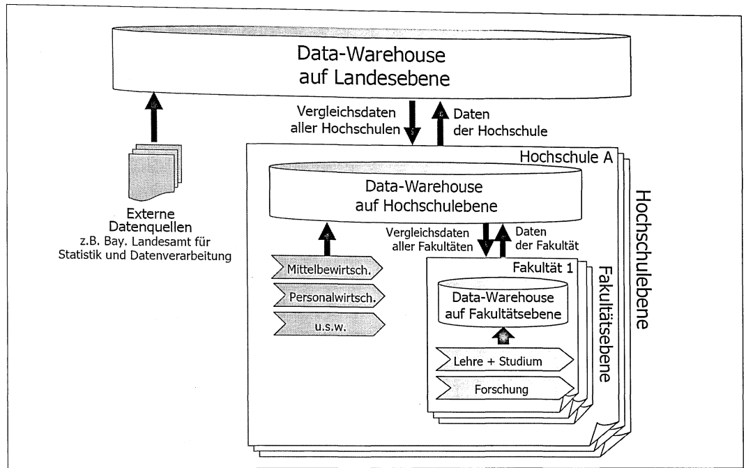
Abb. 3: Architektur des Data-Warehouse-Systems von CEUS
