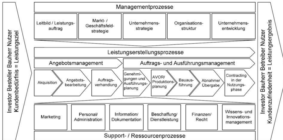
Abbildung 3: Prozessmodell der Wertschöpfungskette eines Bauunternehmens [Girmscheid, 2003]
