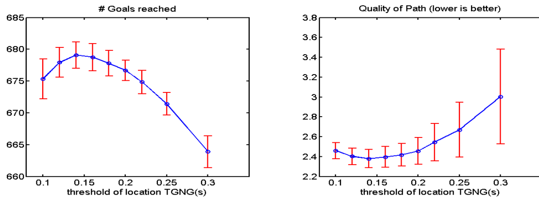
(d) Influence of location space TGNG threshold parameter \theta_L .
