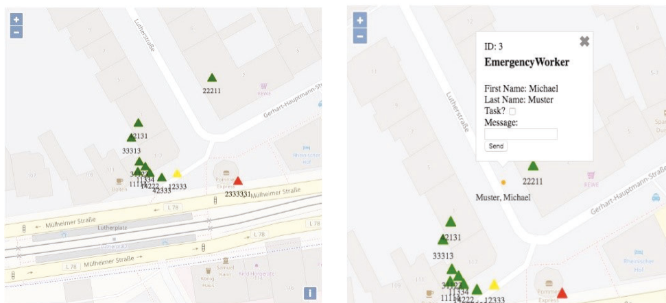
Abbildung 3 – MANVredWeb Ansicht; Beispiel Details Einsatzkraft
