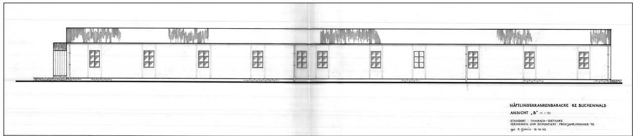
64 Ansicht Baracke Zustand Tambach-Dietharz 1993, Rosemarie Garcia, alle Fenster sind gleich breit dargestellt
