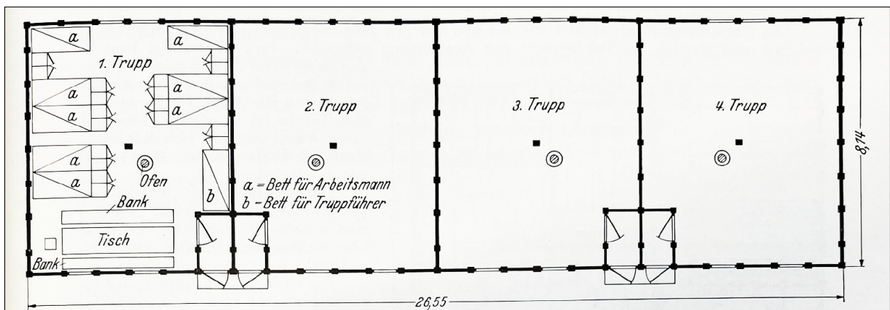
Abb. 2. Mannschaftsbaracke (Typ RL IV) für 4 Trupps.
