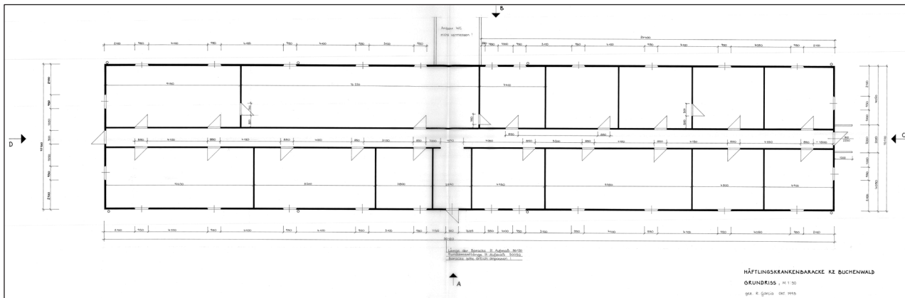
49 Grundriss Baracke Zustand Tambach-Dietharz 1993, Rosemarie Garcia
