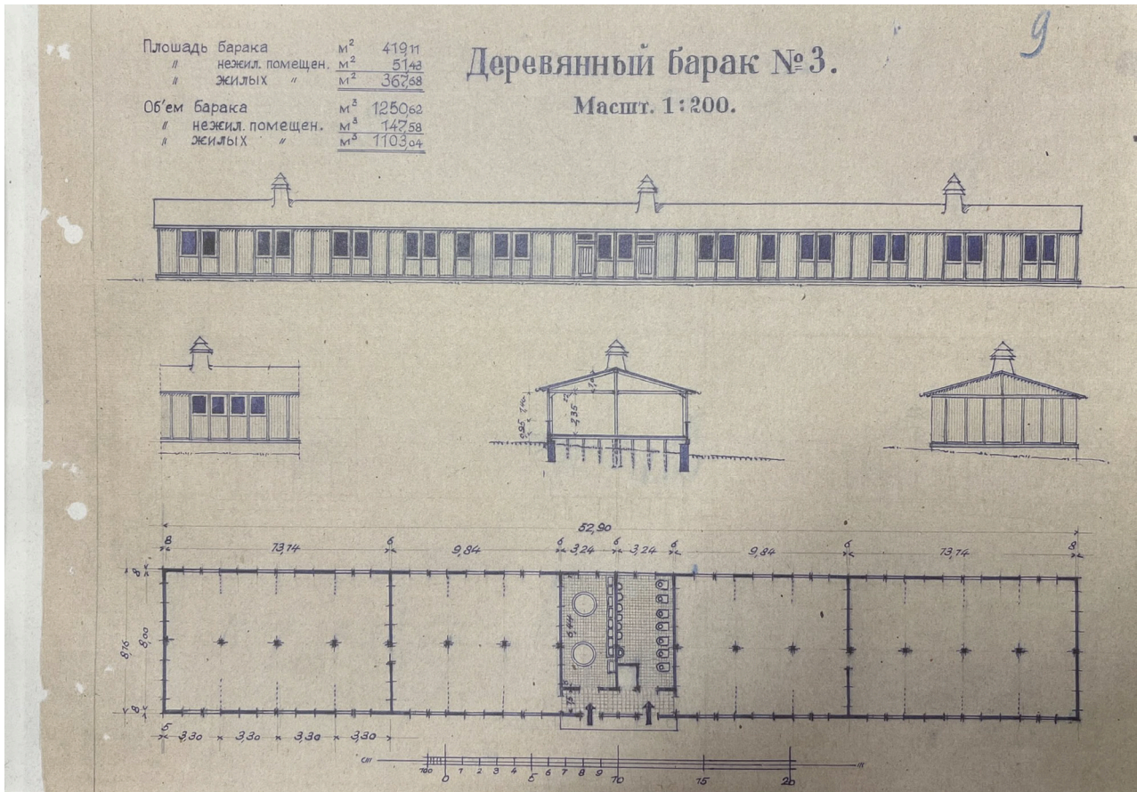
18 RAD-Unterkunftsbaracke in Buchenwald, Zeichnung 1948
