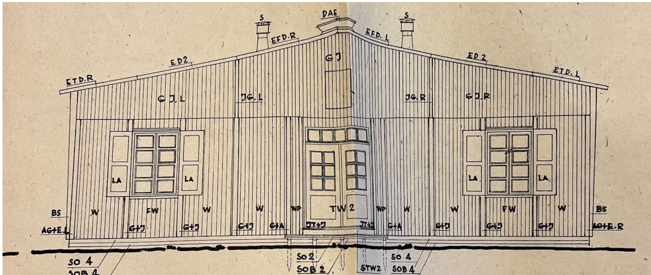
10 BfH-Baracke Typ 20 601 Ansicht
