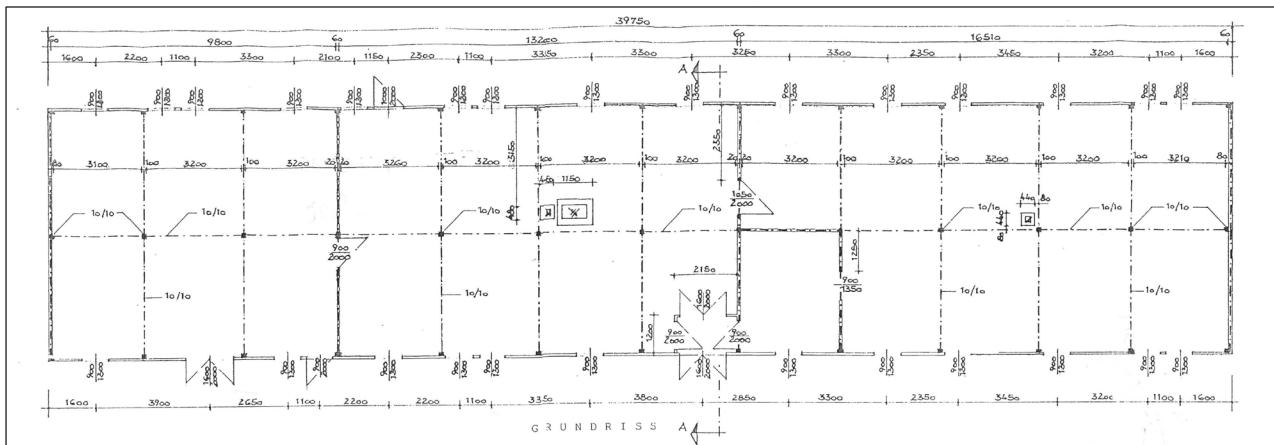
72 Grundriss Tischlereibaracke, KZ-Gedenkstätte Mittelbau-Dora
