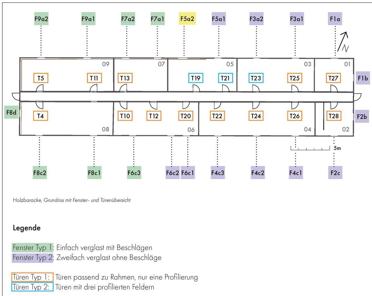
35 Grundriss Baracke, Übersicht Fenster und Türen
