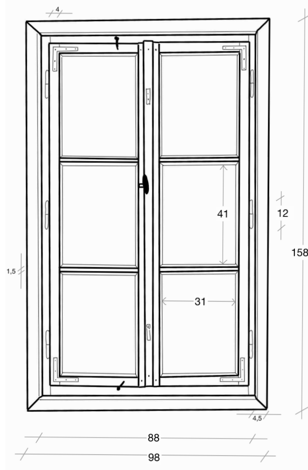
Skizze Fenster Typ 1 innen am Beispiel von F7a2, Maßangaben in cm
