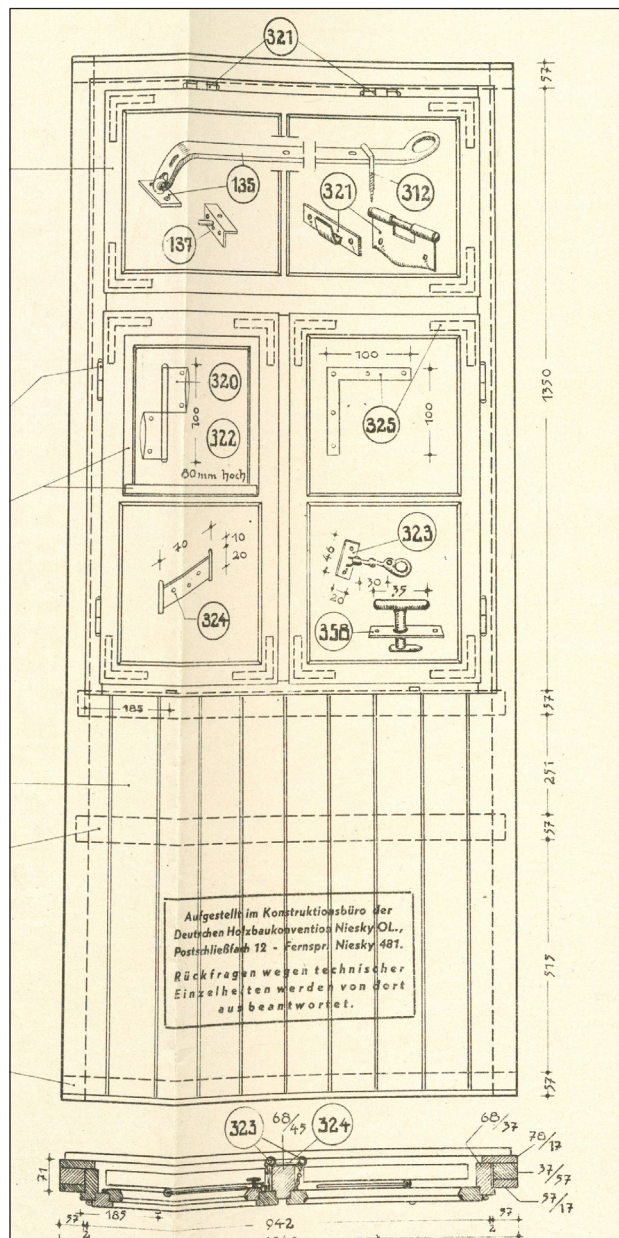
37 BfH-Baracke Typ 20 601 Innentürtafel
