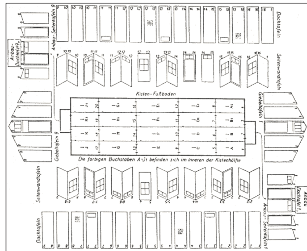
4 Verzeichnis der Bauteile einer Doecker-Normalbaracke, um 1910
