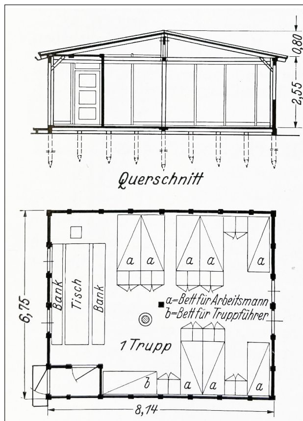
6 Mannschaftsbaracke RL IV, Grundriss eines Mannschaftsmoduls und Querschnitt
