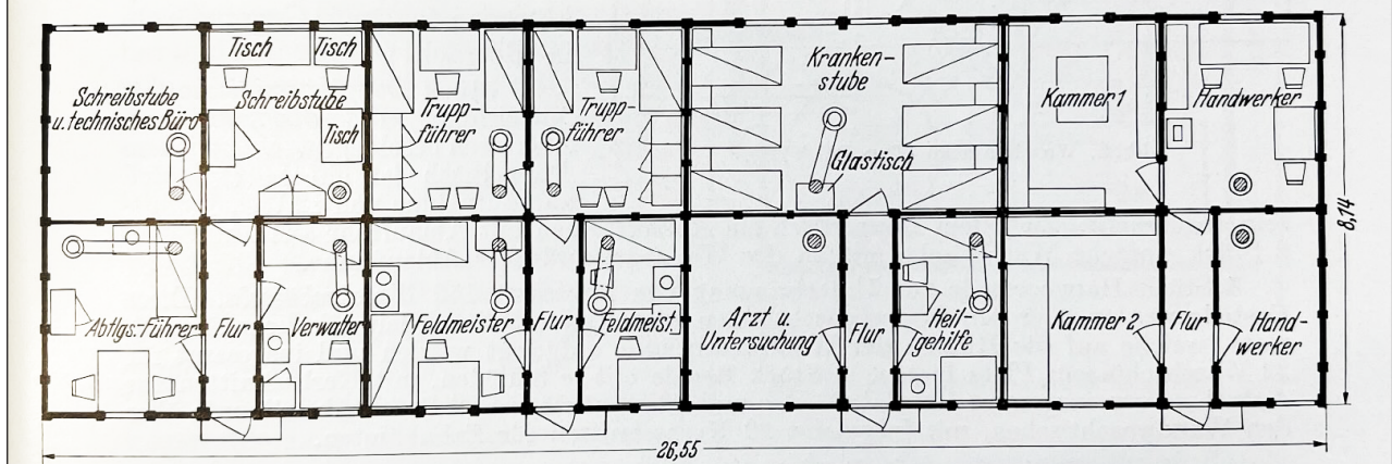
5 Grundrisse Mannschaftsbaracke RL IV (oben) und Verwaltungsbaracke RL V (unten)
