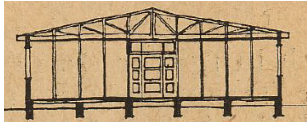
16 Ausschnitt: Schnitt mit Binderkonstruktion Protektoratsbaracke
