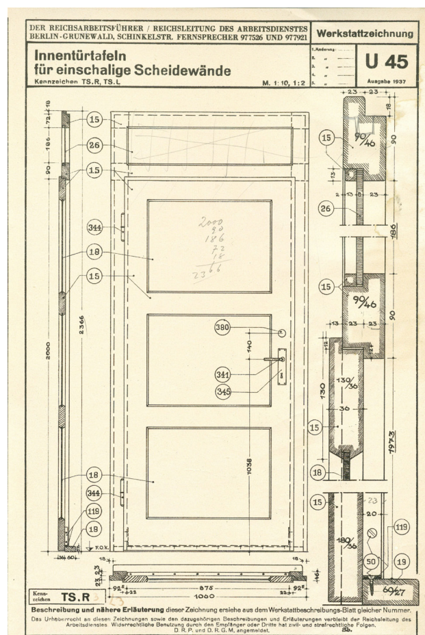
39 RAD-Baracke RL IV Innentürtafel
