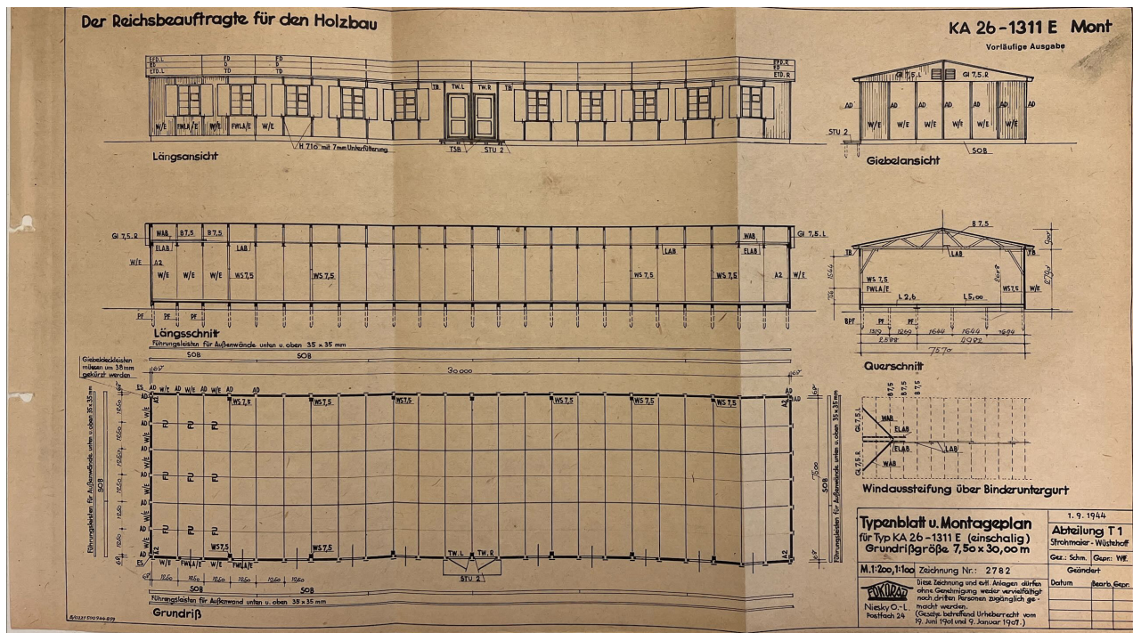
15 Montageplan KA-Baracke 26-1311 E
