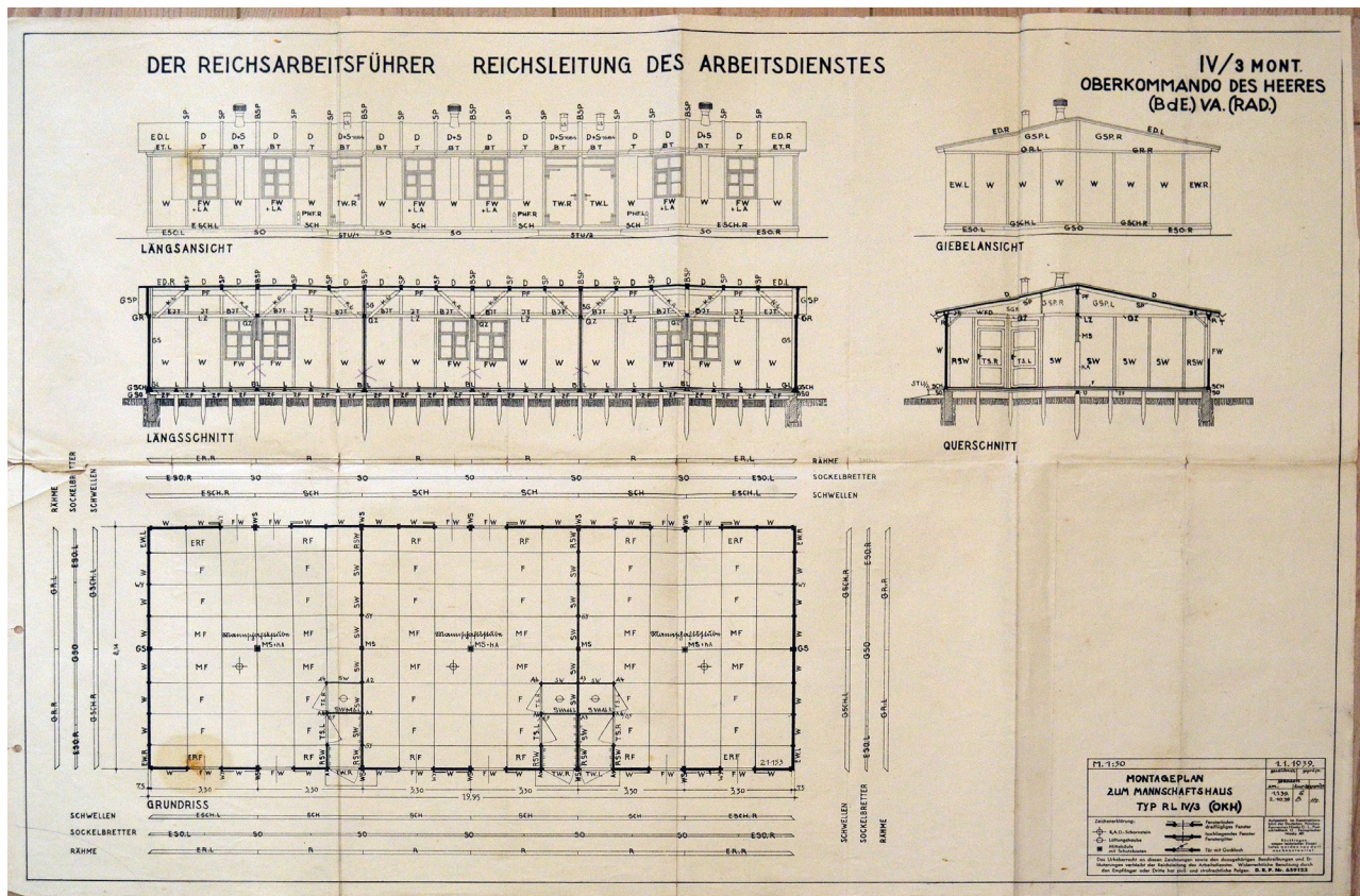
7 Montageplan Mannschaftsbaracke RL IV/3
