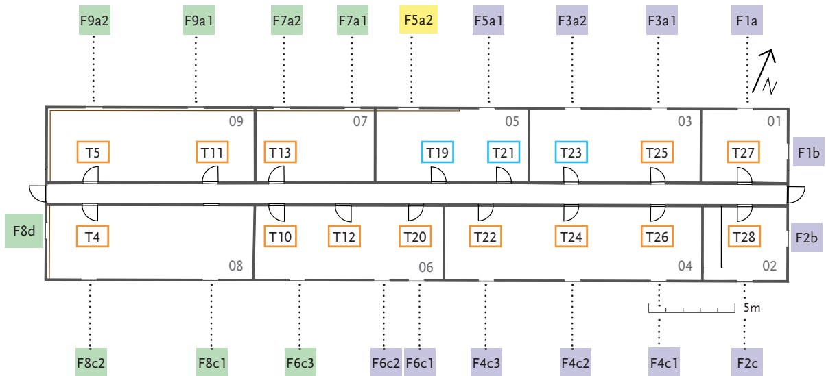
Holzbaracke, Grundriss mit Fenster- und Türenübersicht
