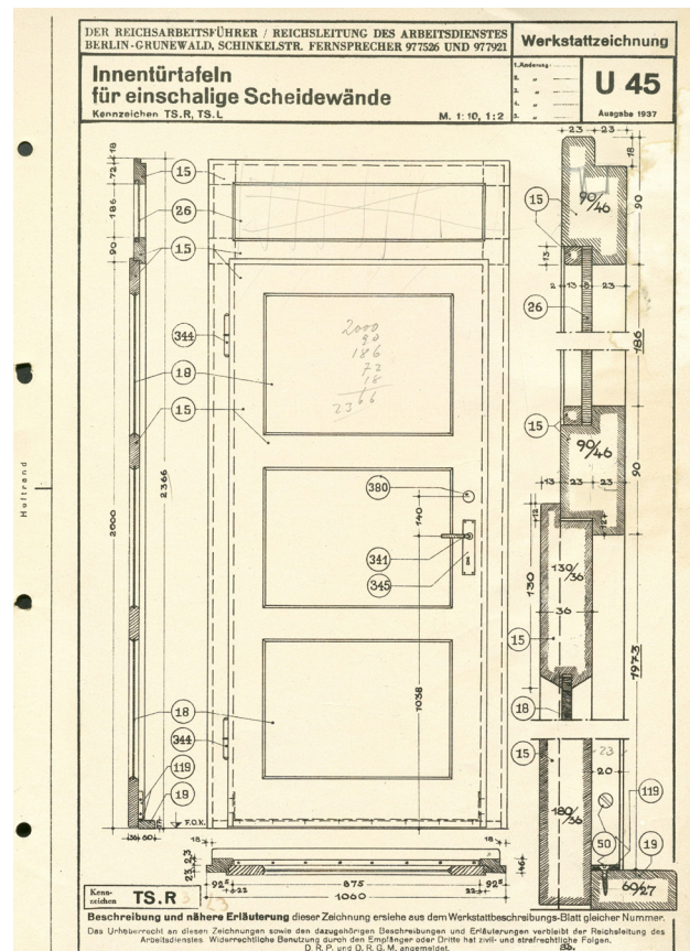
8 Werkstattzeichnung Innentürtafel Typ RL IV
