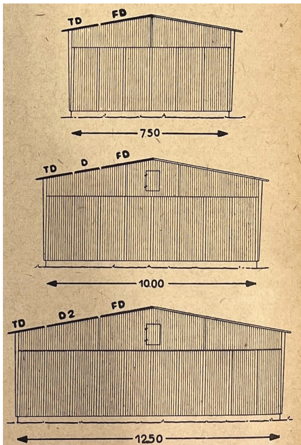
11 Gebäudetiefen der BfH-Baracken
