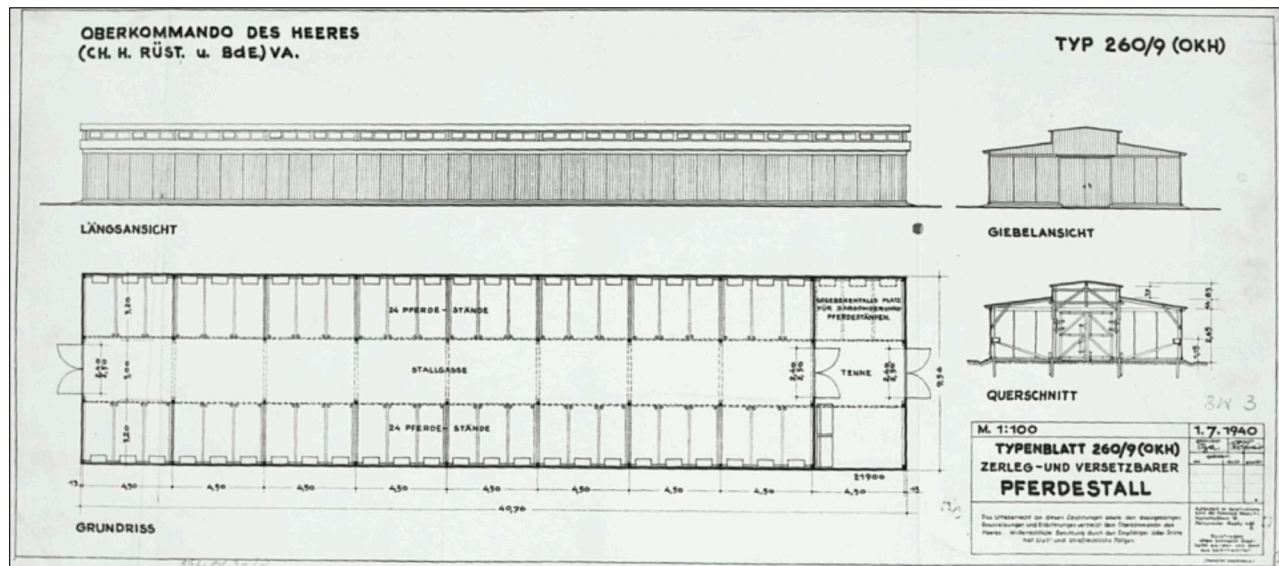
9 Typenblatt 260/9 OKH Pferdestall
