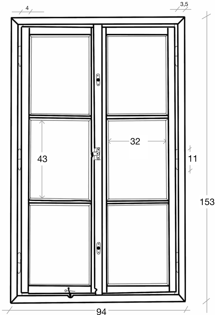
Skizze Fenster Typ 2 innen am Beispiel von F4c1, Maßangaben in cm
