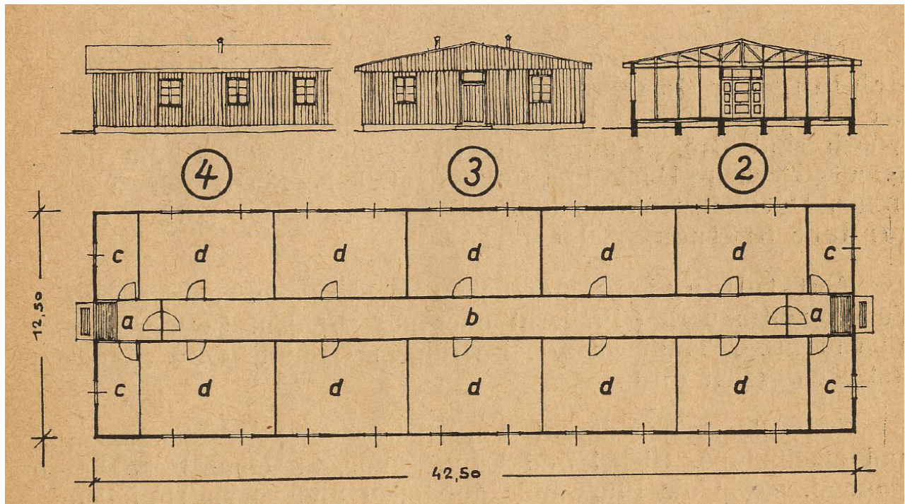
16 Protektoratsbaracke Grundform
