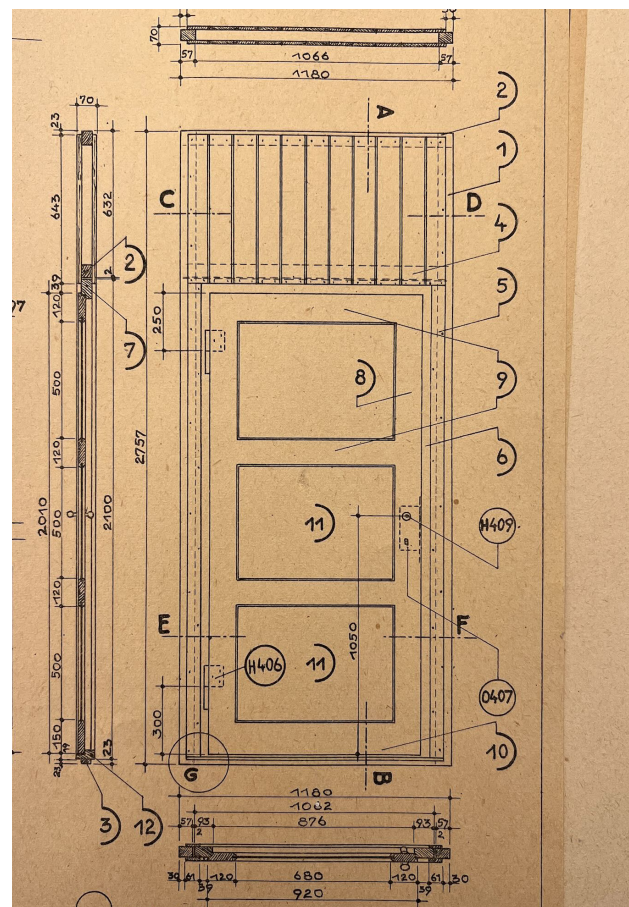
14 BfH-Baracke Typ 20 601 Innentürtafel
