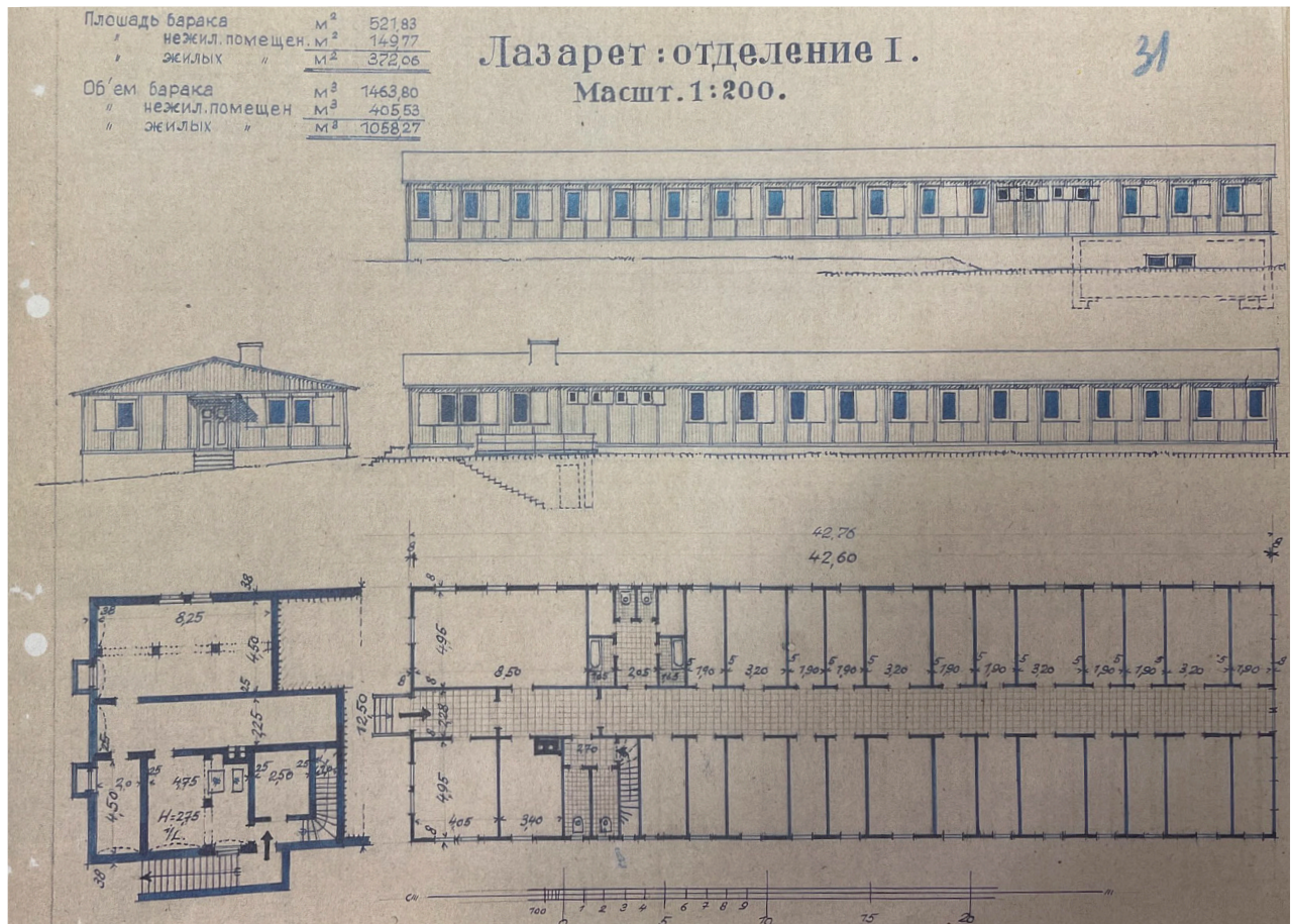
30 Lazarettbaracke in Buchenwald, Zeichnung 1948
