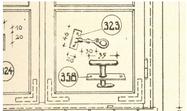
76 RAD-Baracke RL IV/3, Werkstattzeichnung Fensterterafel, Ausschnitt
