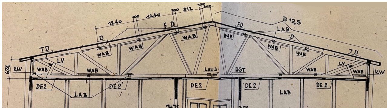
13 Binderstruktur BfH-Baracke Typ 20 601
