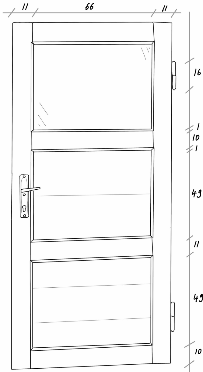
Skizze Türblatt Typ 2 innen am Beispiel von T23, Maßangaben in cm
