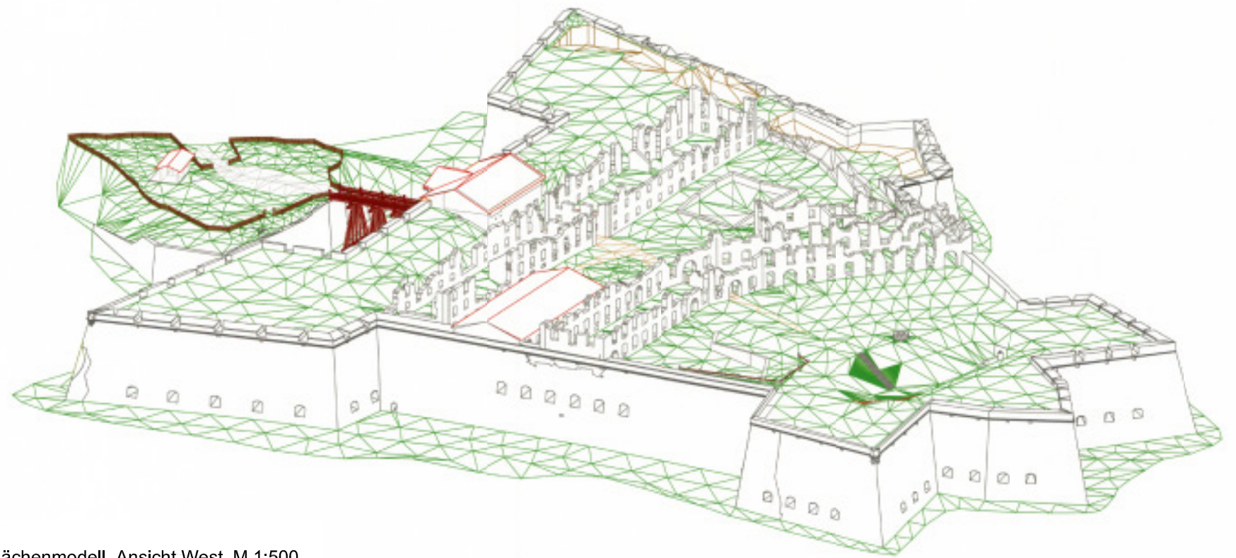
Flächenmodell, Ansicht West, M 1:500
