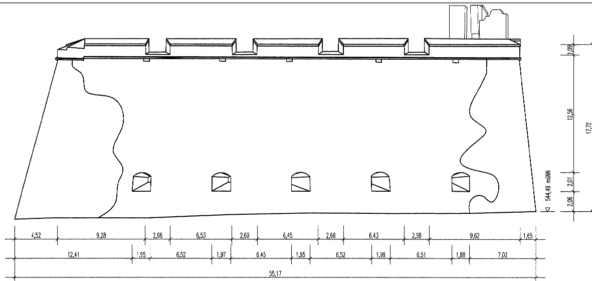
Ansicht 19 Bastion Karl
