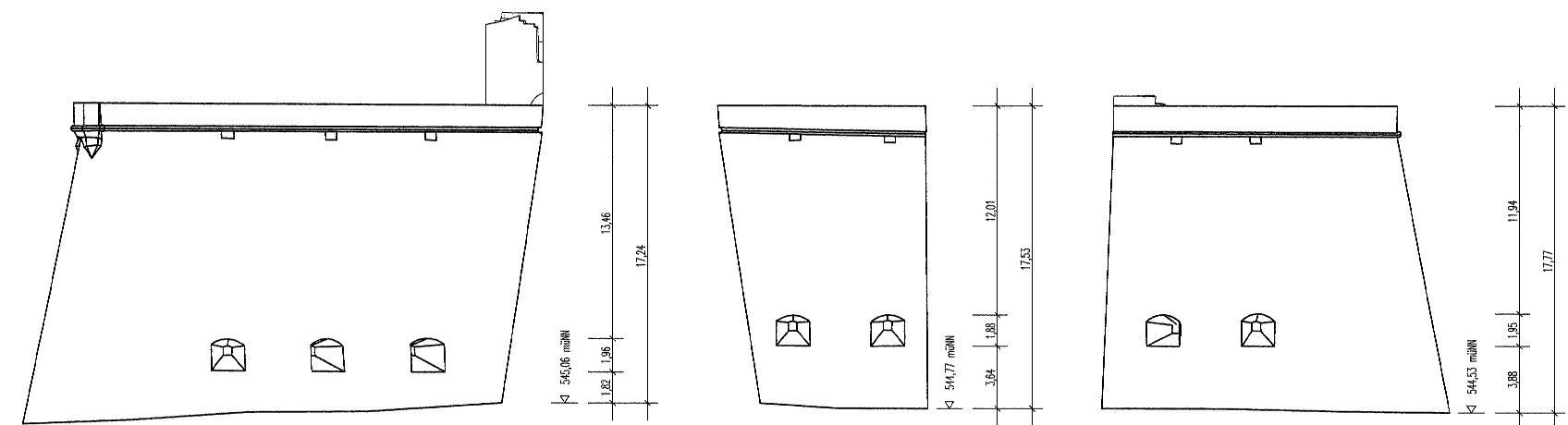
Ansicht 6 Bastion Nürnberg Südostseite
