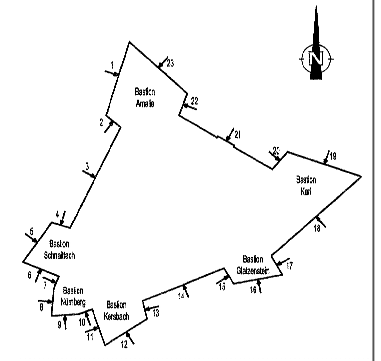
Abwicklung 19 - 23 M 1:200
