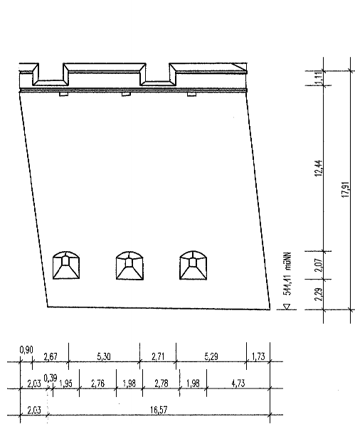
Ansicht 22 Bastion Amalie Ostseite
