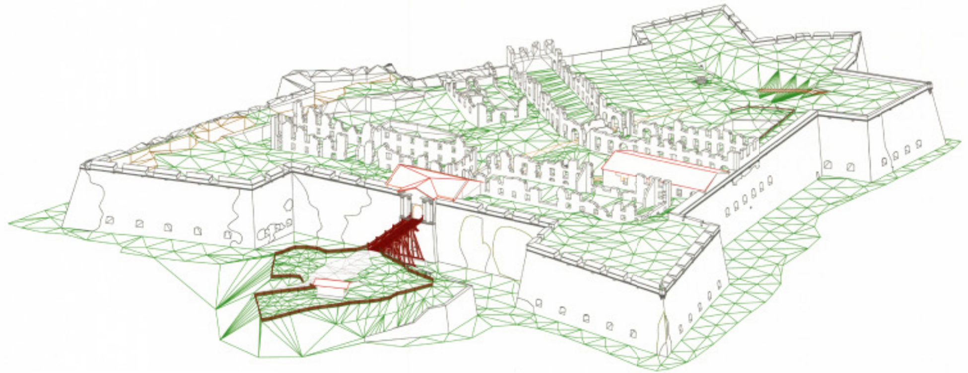
Flächenmodell, Ansicht Nord, M 1:500
