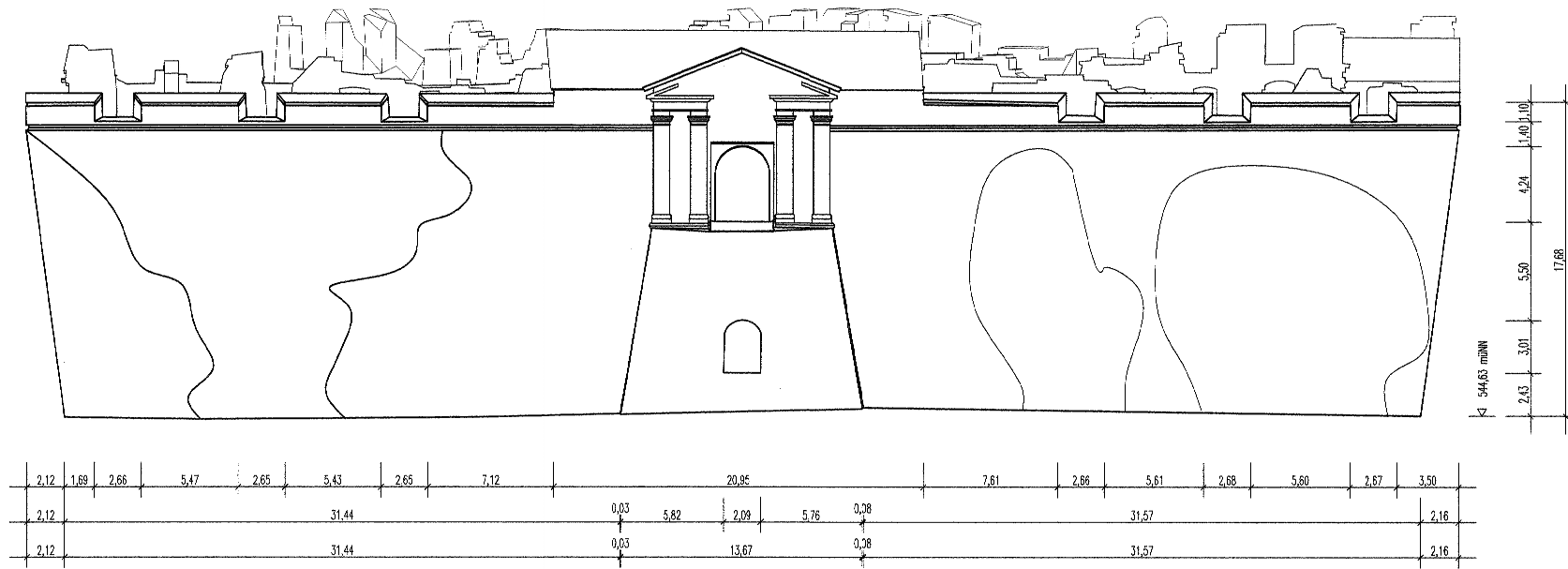
Ansicht 21 Courtine mit Torhaus Nordostseite
