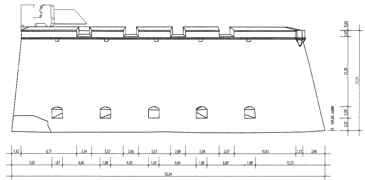
Ansicht 23 Bastion Amalie Nordseite
