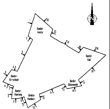
Abwicklung 6 - 11 M 1:200
