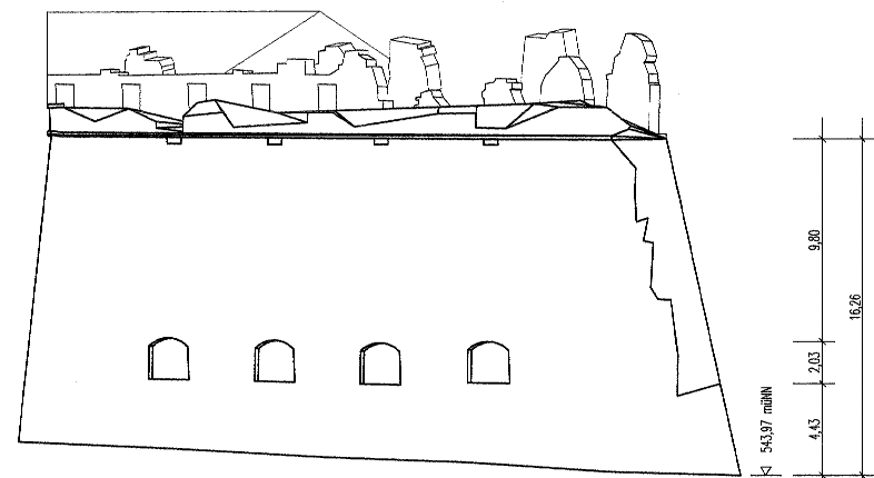
Ansicht 15 Bastion Glatzenstein Westseite
