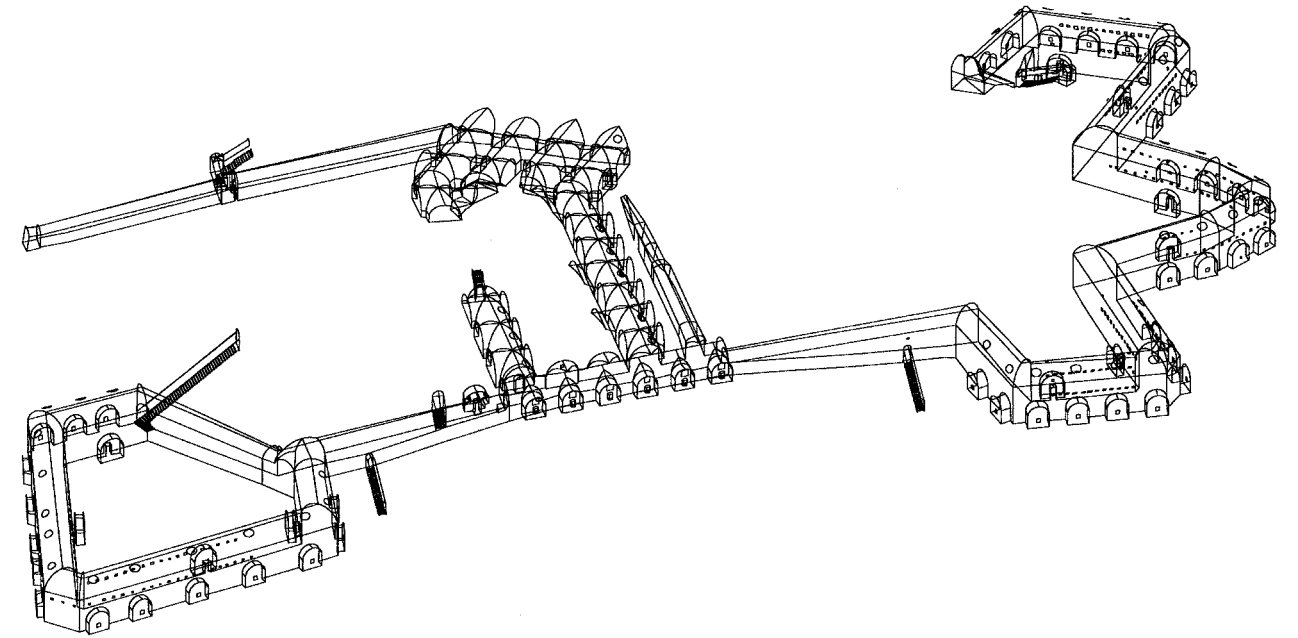
Gittermodell Kasematten, M 1:500
