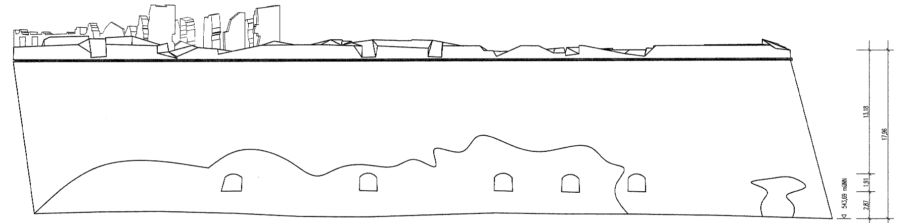
Ansicht 13 Bastion Kersbach Ostseite
