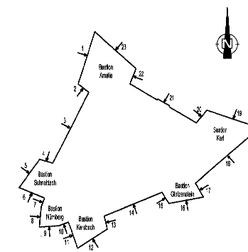
Abwicklung 1 - 5 M 1:200
