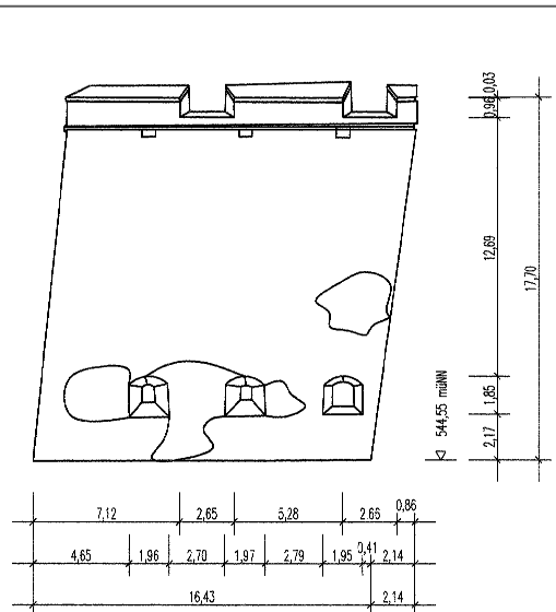
Ansicht 20 Bastion Karl
