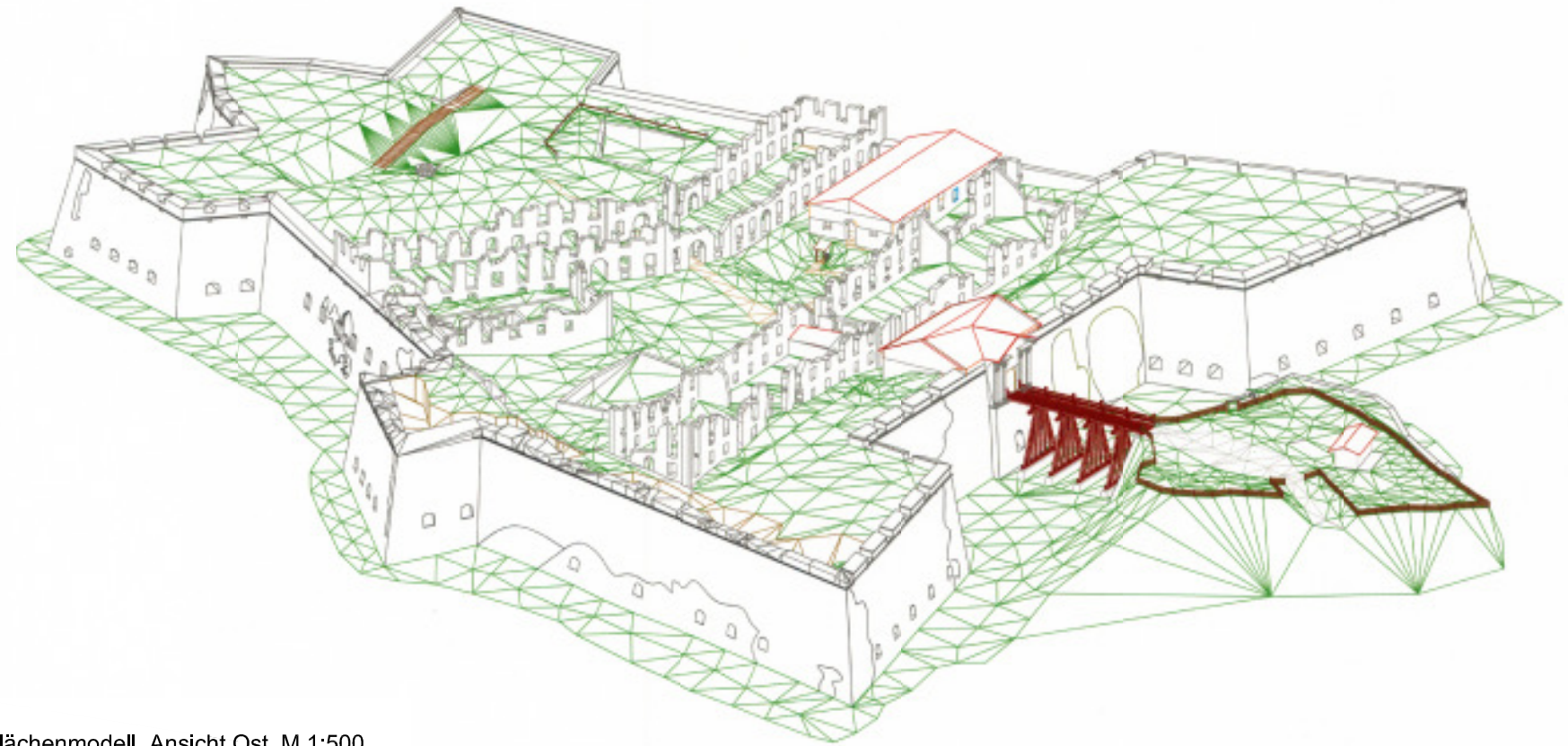
Flächenmodell, Ansicht Ost, M 1:500
