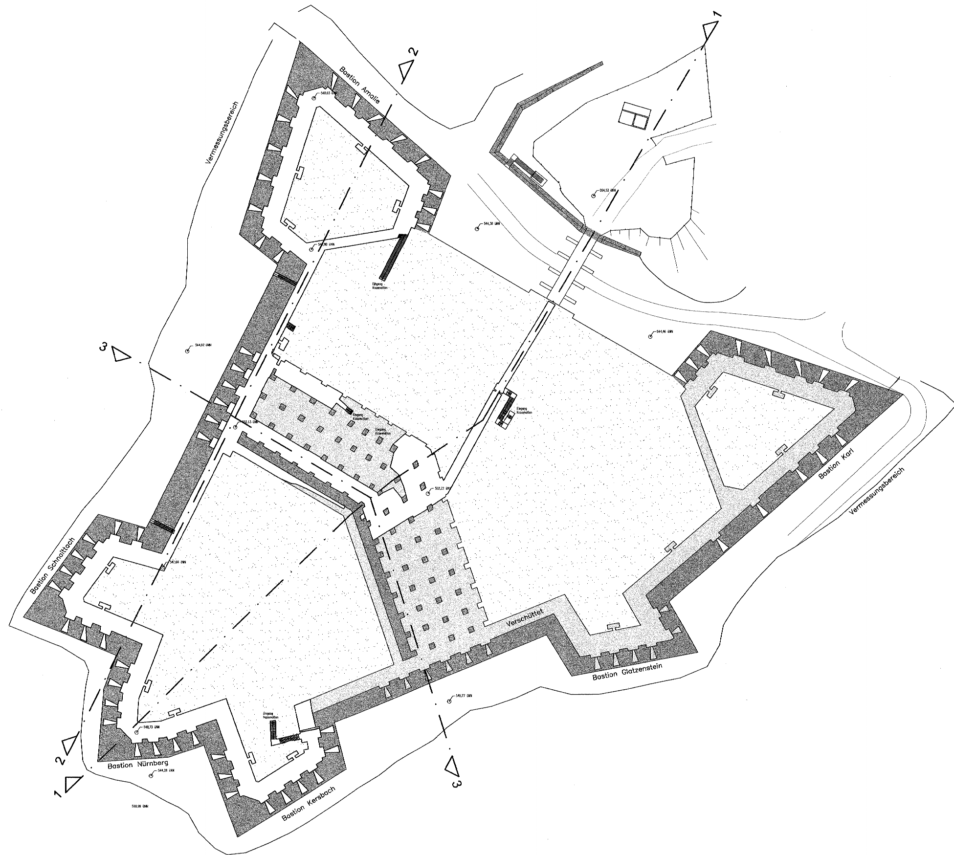
Grundriss Kasematten, M 1:500
