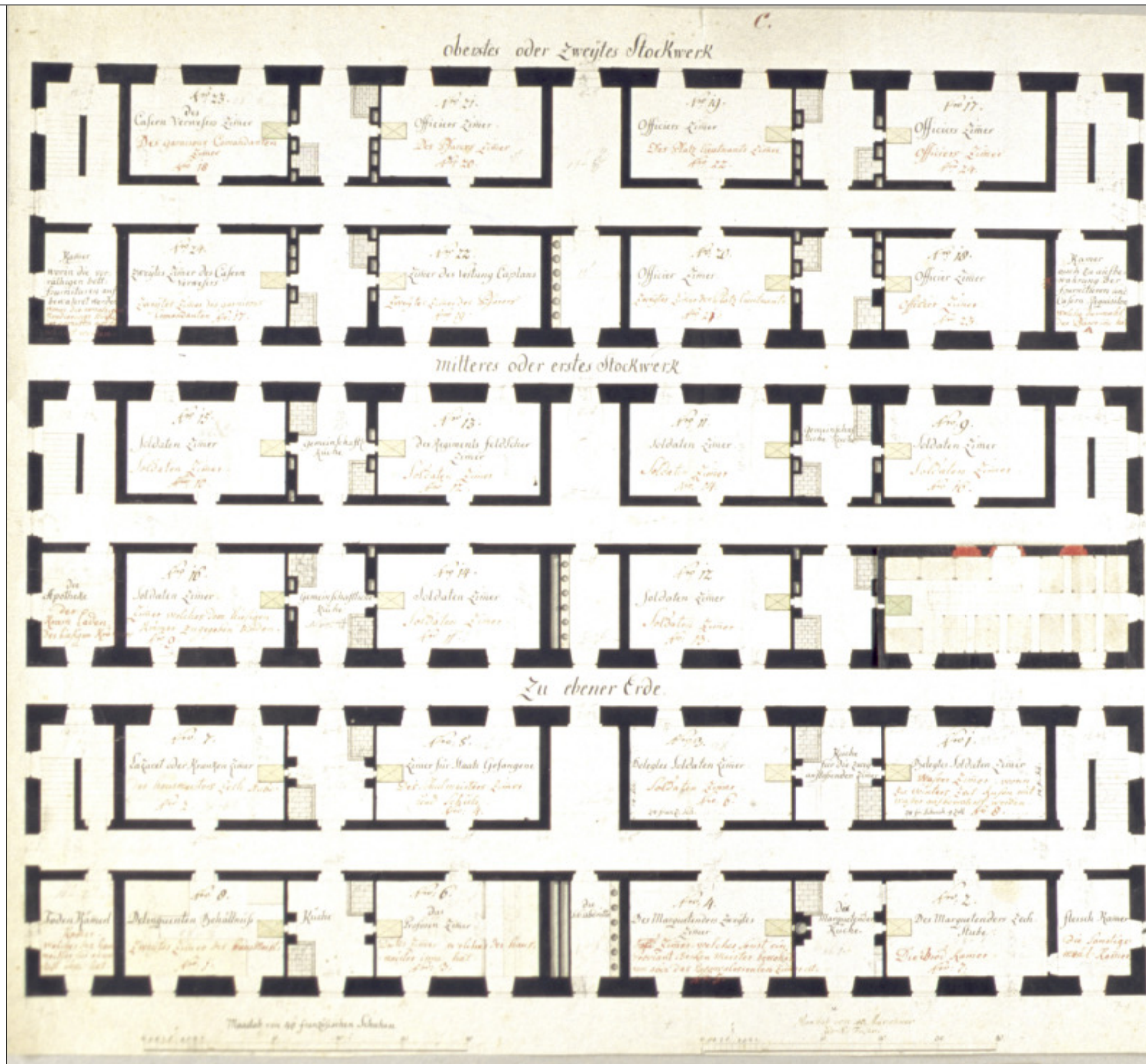
P 026 a um 1750 "Plan Der Rottenbergischen sogenannten alten Caserne", "ebener Erde", "erstes Stockwerk", "zweites Stockwerk" unbekannt Kriegsarchiv München, Plansammlung Rothenberg, Nr. 56
