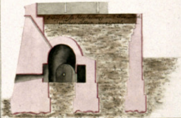
Profil A nach der Linie, a. b.
