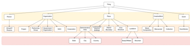
Abbildung 1: Ein Ausschnitt aus dem Zielschema für die Typklassifikation, basierend auf schema.org.
