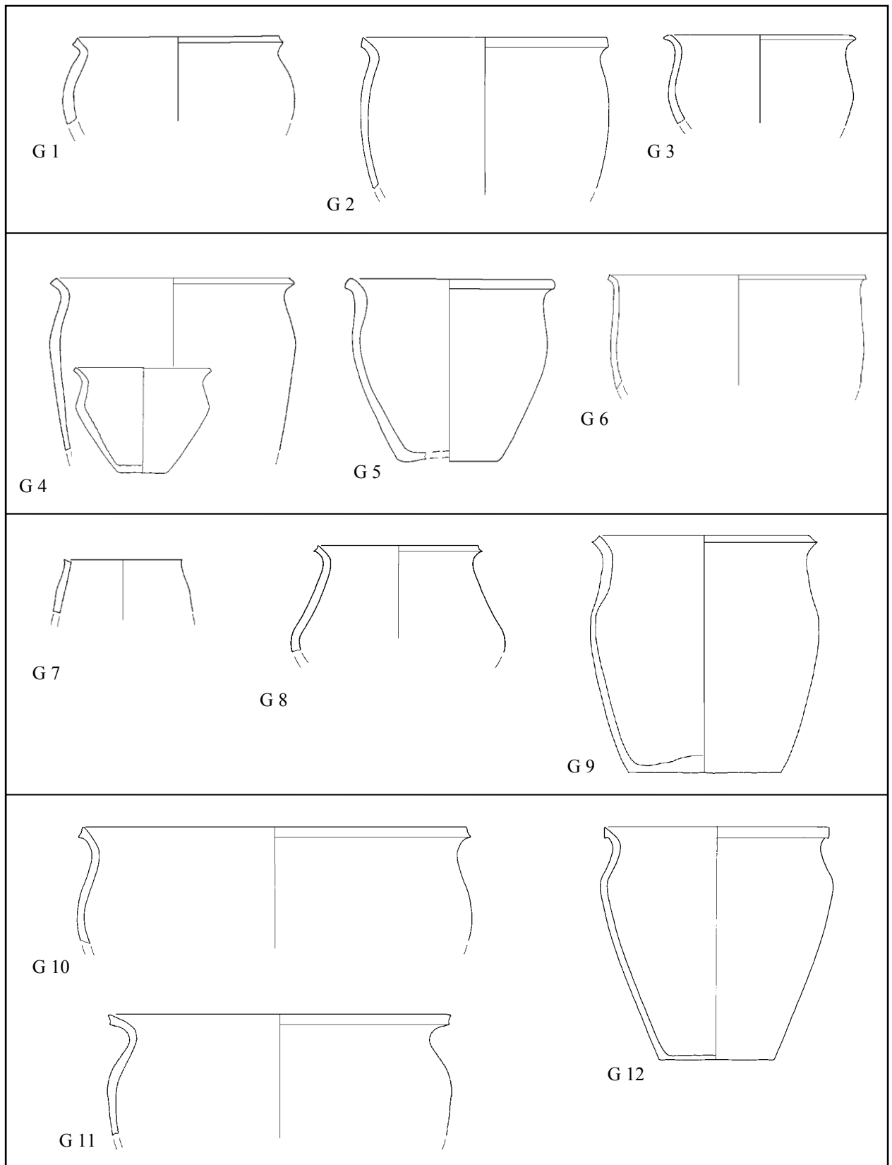
Gefäßformen der Warenart 1, Warenart 2 und Warenart 3 (M 1:5)
