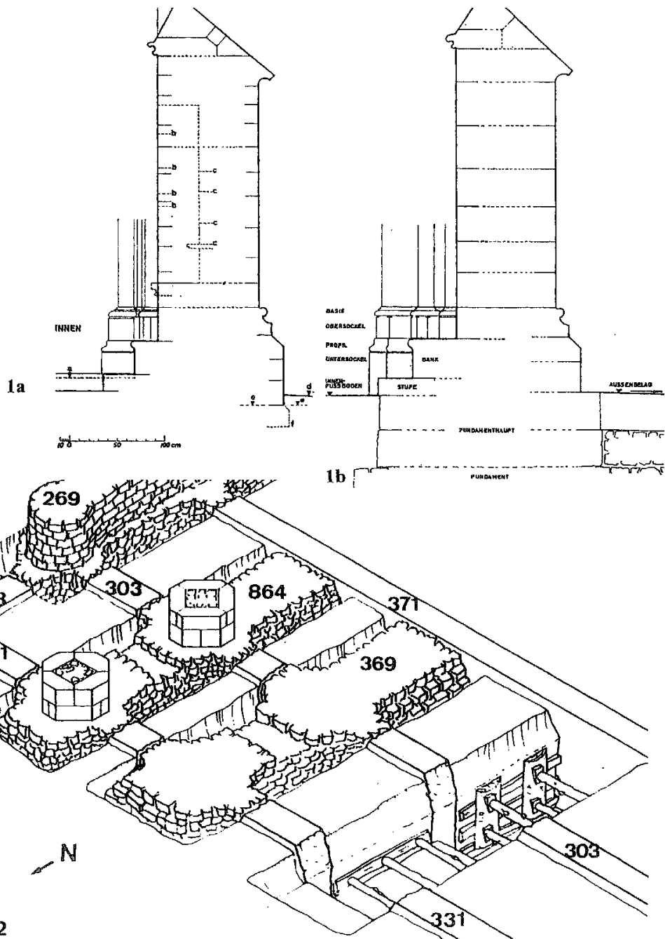
Taf. 54. 1a-b Kölner Dom. Schnitte durch die Außenwand der Agneskapelle zwischen den Pfeilern A 18 1 und A 18 2 (Feld 68) bzw. durch die südliche Außenwand des Langchores zwischen den Pfeilern A 13 und A 14 (Feld 56). a heutiger Fußboden; b Fugen rechts von der Piscina; c Fugen in der Rückwand der Piscina; d Oberkante des Außenbelages; e Oberkante des Fundamentes; f geplante Sockelschräge (nach Wolff 1968). M. 1:50. – 2 Köln, Domgrabung. Isometrische Darstellung der karolingisch-ottonischen (B331, B303, B371) und der gotischen Fundamente (B269, B864, B369) in den südlichen Langchor-Seitenschiffen während der Errichtung, Blickrichtung von Nordwesten (nach Wolff 1986b, verändert).
