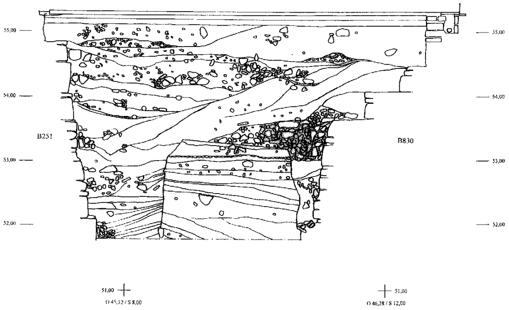
Taf. 52a. Köln, Domgrabung. Profile SO-NW (Z695) und NW-SO (Z696) in Schnitt B270 mit den Baugruben für die Chorpfeiler B 20 (B830) und C 20 (B251). M. 1:50.
