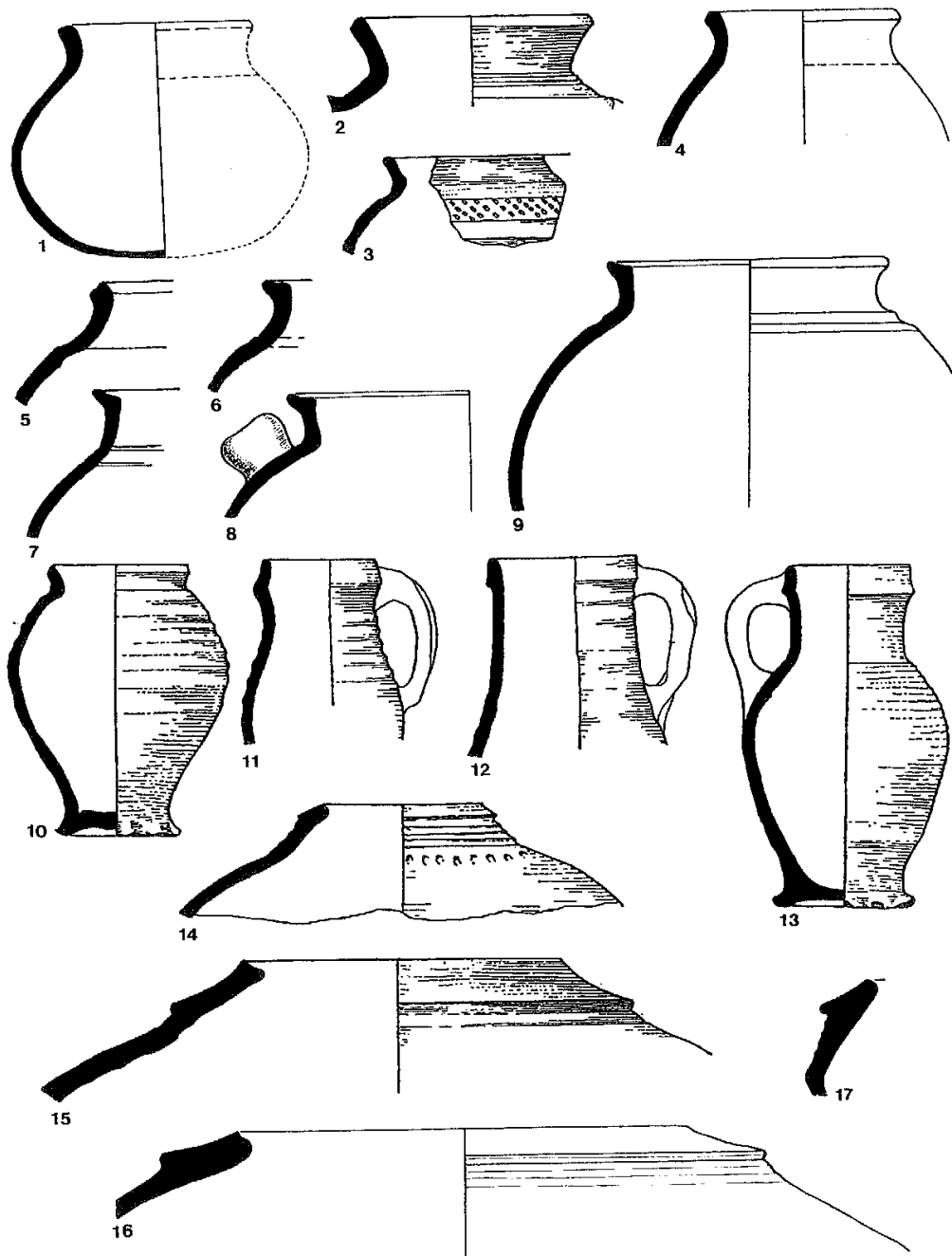
Taf. 41. Morken (ehem. Stadt Bedburg, Erftkreis). Keramik aus Grubenhaus C (nach Hinz 1962a bzw. Hinz 1969a, verändert). M. 1:3.
