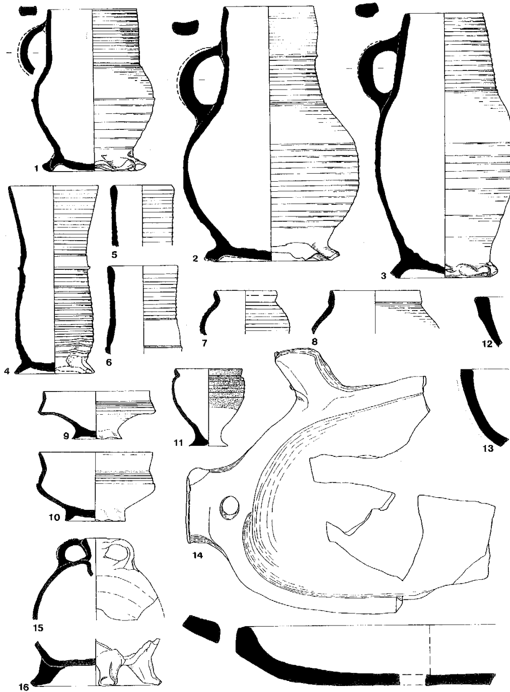
Taf. 43. Köln, Dom. Keramik aus den gotischen Baugruben in den südlichen Langhaus-Seitenschiffen (ca. 1330): 1-11.15 Steinzeug; 12-14.16 Glasierte Irdenware (nach Hauser 1990b, verändert). M. 1:3.
