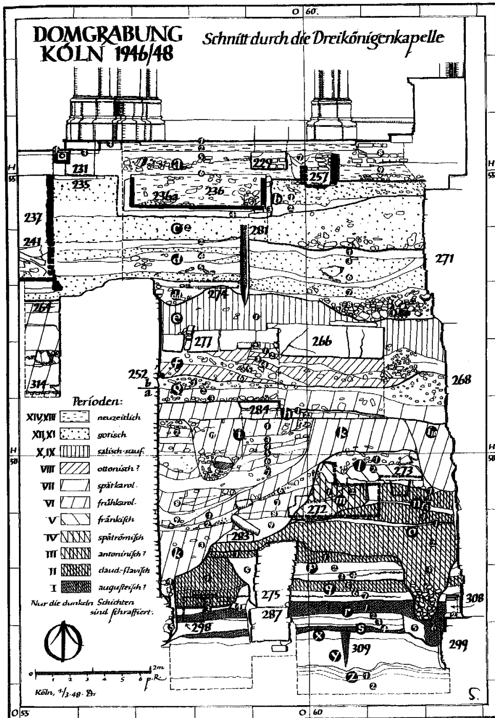
Taf. 49. Köln, Domgrabung. W-O-Profil B280 (Z743) in der Achskapelle (nach Doppelfeld 1948c). M. ca. 1:75.
