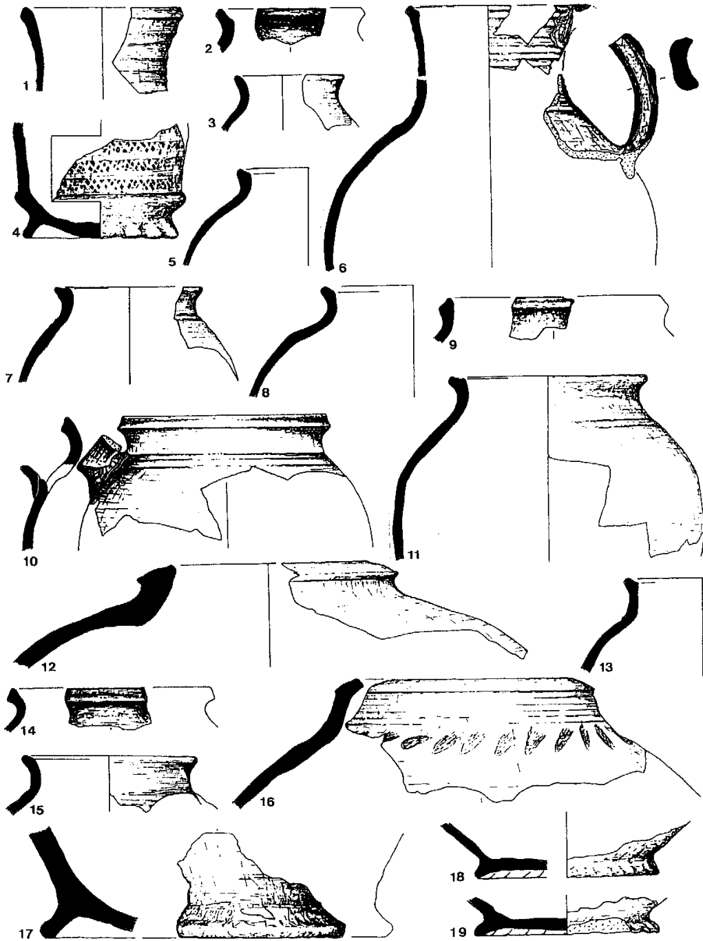
Taf. 33. Königshoven (chem. Stadt Bedburg, Erftkreis; FR 96), Keramik aus Grubenhaus 98: Graue Irdenware (nach Bauche 1997, verändert). M. 1:3.
