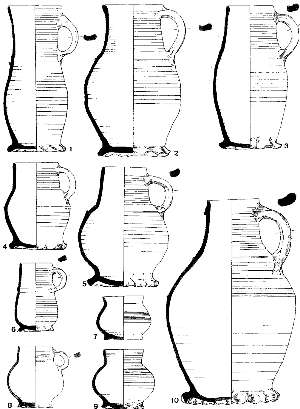
Taf. 23. Siegburg (Rhein-Sieg-Kreis), Scherbenhügel Aulgasse. Steinzeugformen der frühen Periode 4 (nach Beckmann 1975, verändert; Zusammenstellung nach Angaben bei Hänel 1987a bzw. 1987b). M. 1:3.
