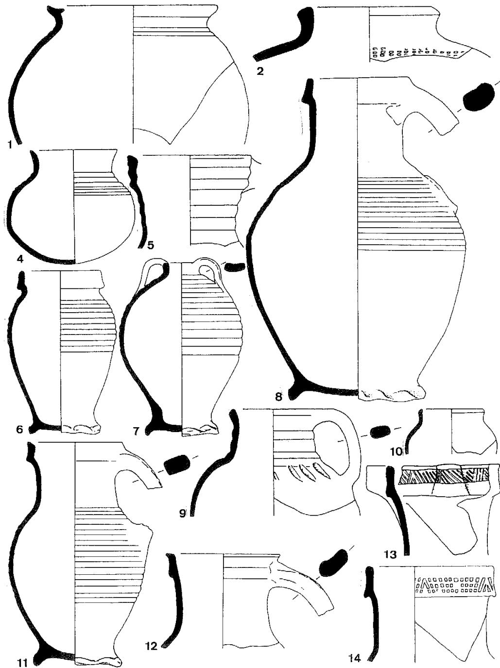
Taf. 26. Meckenheim (Rhein-Sieg-Kreis), Töpfereiabfälle: Protosteinzeug (nach Stilke 1996, verändert). M. 1:3.
