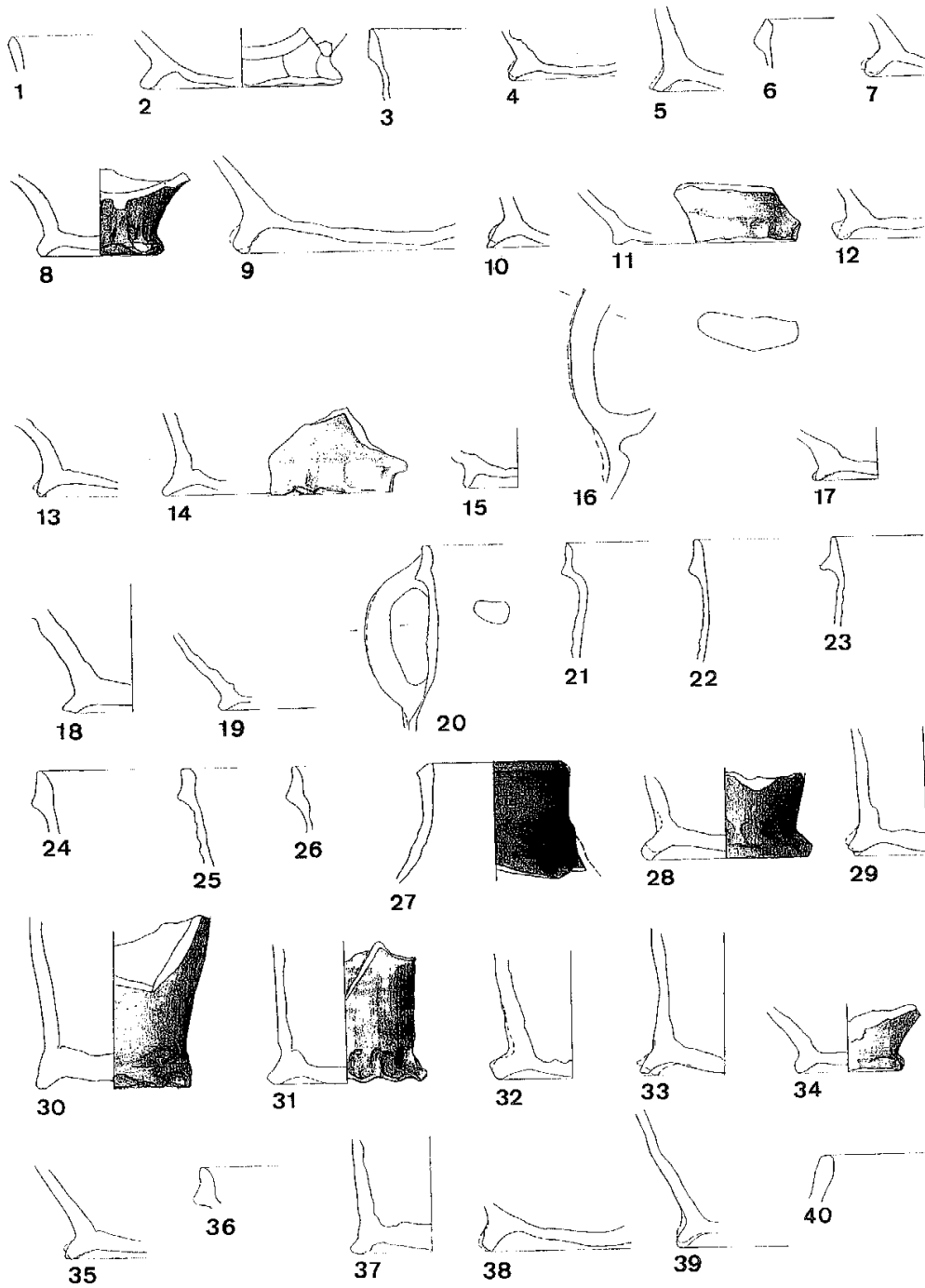
Taf. 8. Domgrabung Köln. Oxidierend gebrannte Irdenwaren (1 W 1; 2 W 2; 3-5 W 4; 6-12 W 5; 13-15 W 6; 16-18 W 7; 19 W 8; 20-21 W 9; 22-24 W 10; 25-35 W 11; 36-38 W 12; 39 W 14; 40 W 15). M. 1:3.
