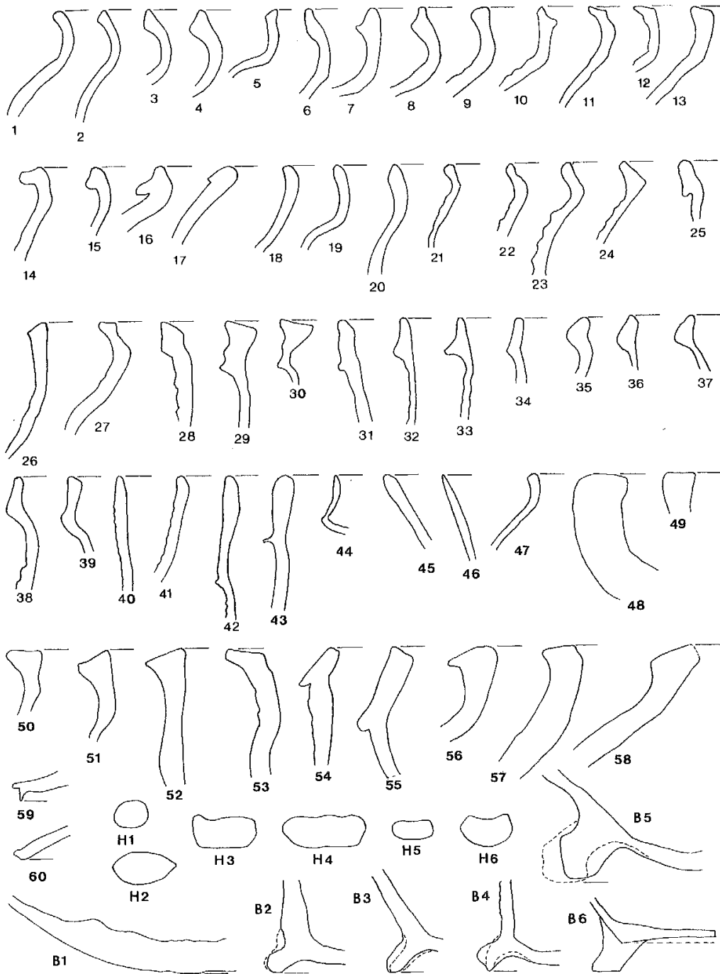
Taf. 7. Domgrubung Köln. Typen der Randformen, der Handhaben und der Bodenformen/Standvorrichtungen der spätmittelalterlichen Keramik. M. 1:2.
