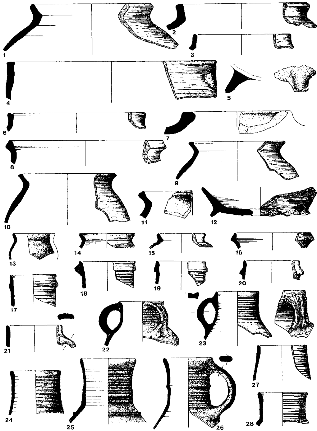
Taf. 38. Duisburg, Alter Markt. Keramik aus Schicht 4: 1-12 Graue Irdenware; 13-28 Protosteinzeug bzw. Faststeinzeug (nach Krause 1983a, verändert). M. 1:3.
