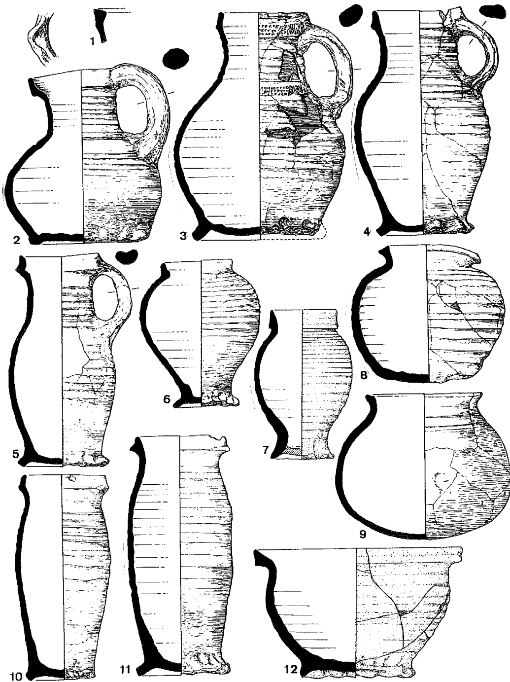
Taf. 40. Neuss. Ausgewählte Keramik aus der Grube am Quirinusstift: 1-11 Protosteinzeug; 12 Graue Irdenware (nach Sommer 1987, verändert). M. 1:3.
