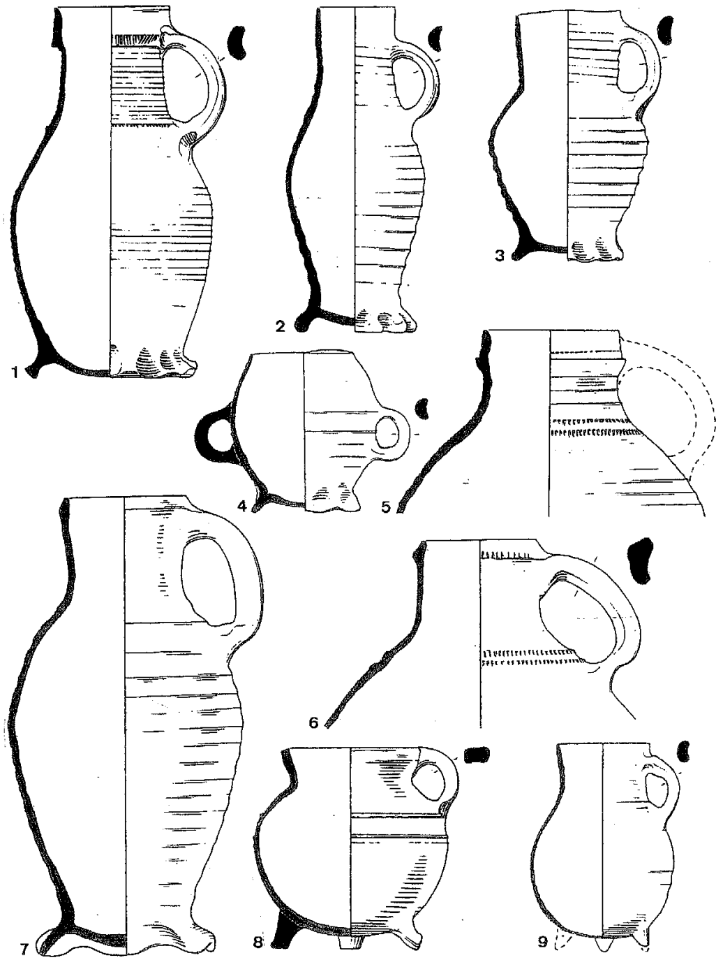
Taf. 27. Langerwiche (Kreis Aachen), Töpfereiabfälle. 1-9 Steinzeug; 8-9 Glasierte Irdenware (nach Hurst 1977, verändert). M. 1:3.
