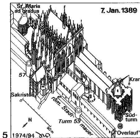
Taf. 45. Kölner Dom. Isometrische Darstellung verschiedener Bauzustände, Blickrichtung von Nordwesten (nach Wolff 1995b).
