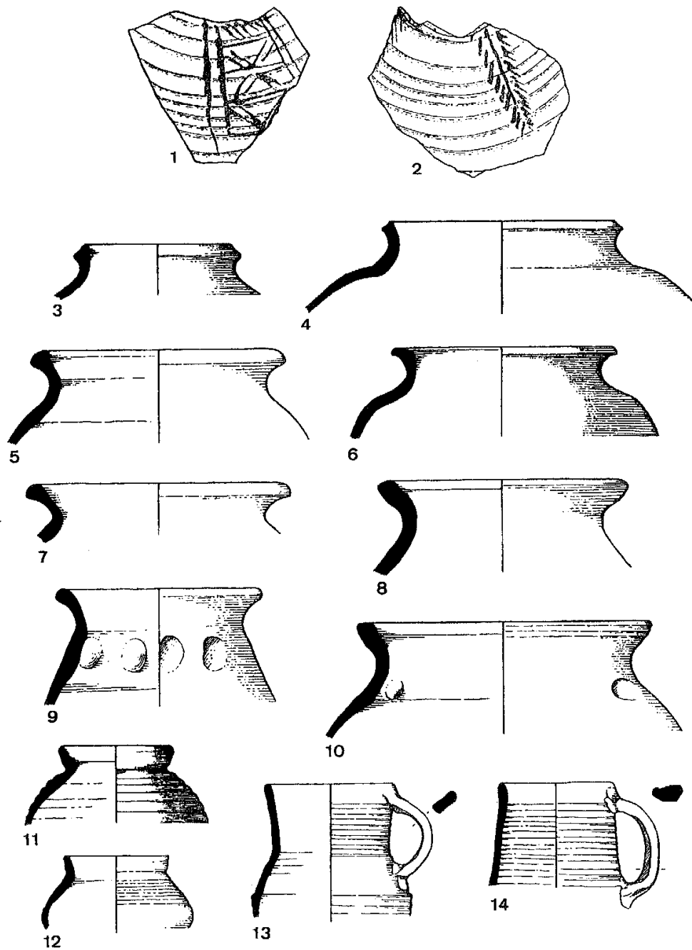
Taf. 35. Burg Alt-Hochstaden (ehem. Grevenbroich-Frimmersdorf, Kreis Neuss), Keramik aus dem Zerstörungshorizont über Schicht III D: 1-2 Oxidierend gebrannte Irdenware mit rotbrauner Bemalung; 3-10 Graue Irdenware; 11-14 Protosteinzeug (nach Herrnbrödt 1958, verändert). M. 1:3.
