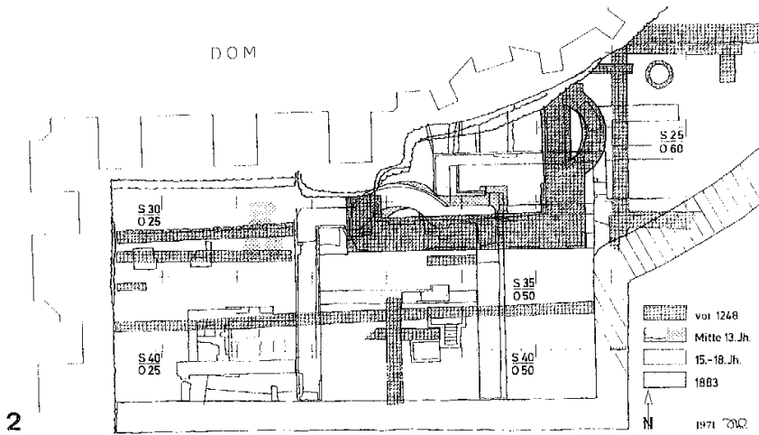
Taf. 53. Köln, Domgrabung. 1 Grundriß des Chores mit dem Stollen B311 und den Grüften im südöstlichen Umgang (nach Weyres 1979/80). M. 1:500. – 2 Befunde südlich des gotischen Langchores mit der Pfalzkapelle St. Johannes in curia (nach Wolff 1971a). M. 1:400.
