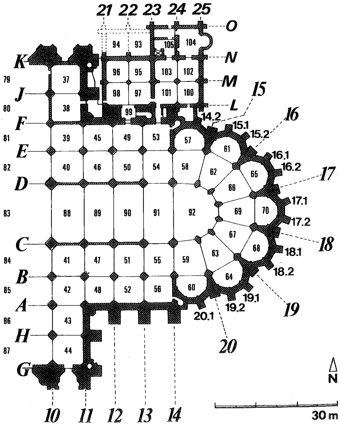
Taf. 3. Kölner Dom. Schematischer Grundriß der Ostteile mit den Nummern der Gewölbefelder und den Bezeichnungen der Pfeiler (nach Arnold Wolff). M. 1:500.
