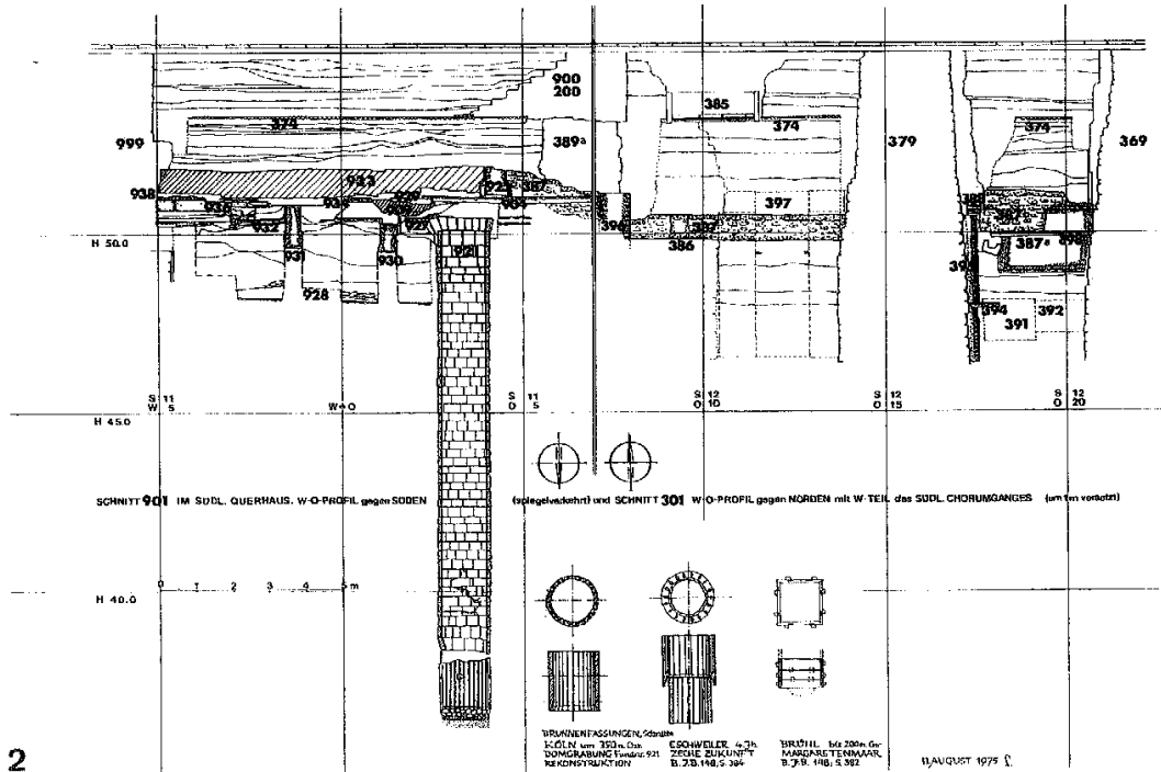
Taf. 55. Köln, Domgrabung. Befunde im südlichen Querhaus und in den südlichen Seitenschiffen des gotischen Domes (nach Weyres 1975, mit Ergänzungen durch den Verfasser). M. 1:200.
