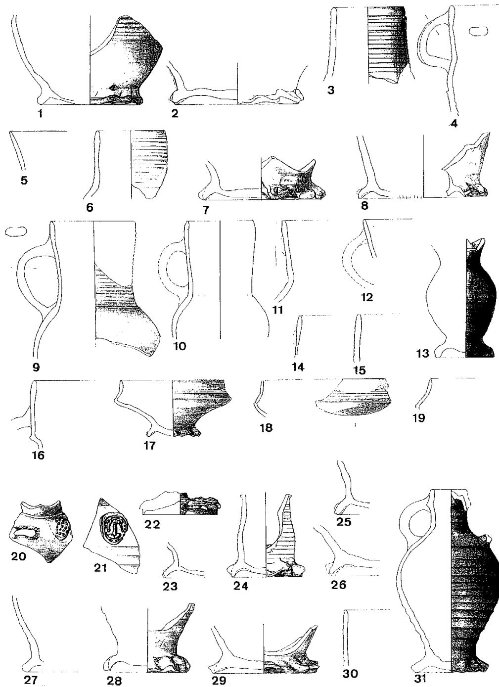
Taf. 14. Domgrabung Köln. Faststeinzeuge (1 W 58; 2 W 59; 3 W 60) und Steinzeuge (4-5 W 61; 6-8 W 62; 9-29 W 64; 30 W 65; 31 W 66). M. 1:3.
