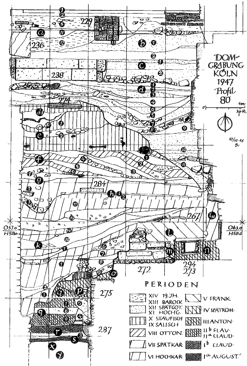
Taf. 50. Köln, Domgrabung. W-O-Profil B80 (Z916/Z917) in der Achskapelle (nach Doppelfeld 1950a). M. 1:50.
