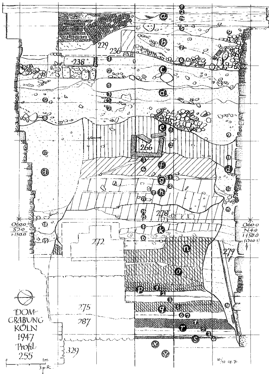
Taf. 51. Köln, Domgrabung. S-N-Profil B255 (Z741/Z742) in der Achskapelle (nach Doppelfeld 1950a). M. 1:50.
