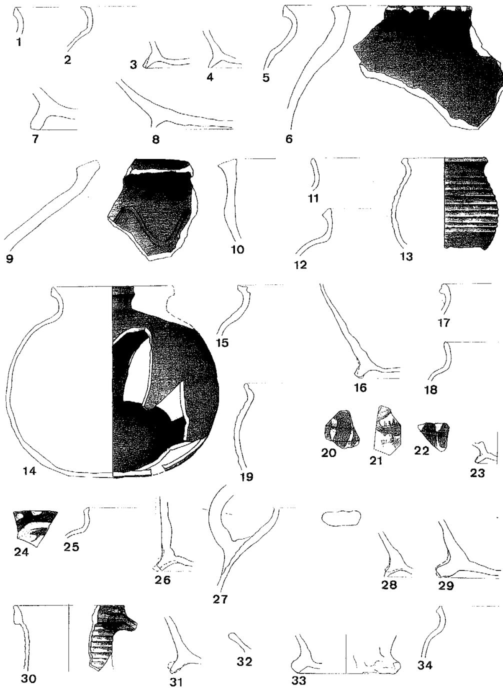
Taf. 10. Domgrabung Köln. Reduzierend gebrannte Irdenwaren (1-4 W 24; 5 W 25; 6 W 26; 7 W 28; 8-10 W 29; 11 W 30; 12-16 W 31) und Protosteinzeuge (17-23 W 32; 24 W 34; 25 W 35; 26 W 36; 27-29 W 37; 30-34 W 39). M. 1:3.
