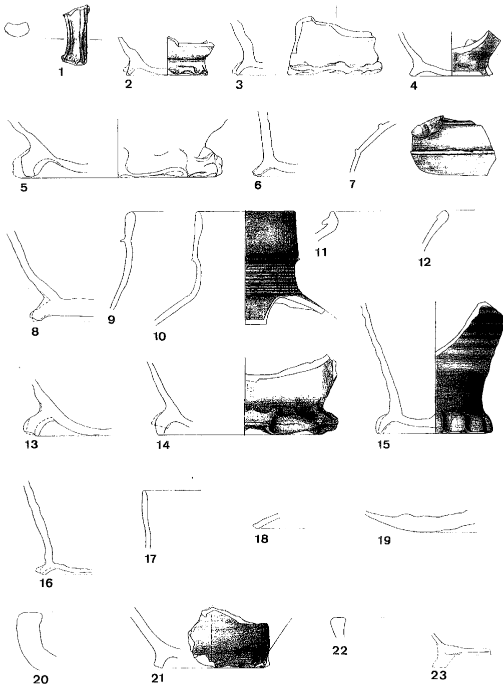
Taf. 15. Domgrabung Köln. Steinzeuge (1-3 W 66; 4 W 67; 5-6 W 68; 7-8 W 69; 9-15 W 70; 16 W 72; 17-18 W 74; 19 W 76) und Glasierte Irdenwaren (20 W 77; 21 W 79; 22 W 80; 23 W 82). M. 1:3.
