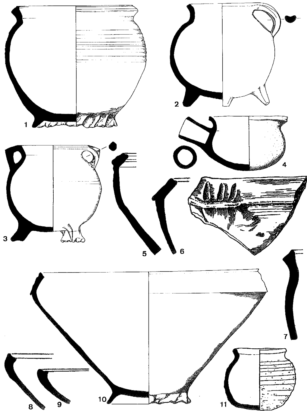
Taf. 29. Brüggcn, Öbel und Overhetfeld (Kreis Viersen), Töpfereiabfälle von verschiedenen Fundstellen (nach Bonner Jahrbücher 146, Locwe 1971 und Rech 1982, verändert). M. 1:3.
