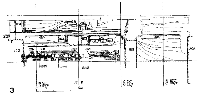
Taf. 57. Köln, Domgrabung. 1 W-O-Profil in der Domachse, Vierung und Binnenchor (nach Doppelfeld 1963). – 2 W-O-Profil etwas nördlich der Domachse, Binnenchor (nach Weyres 1971a). – 3 N-S-Profil, Binnenchor, Feld 91 (nach Weyres 1971a). M. 1:200.
