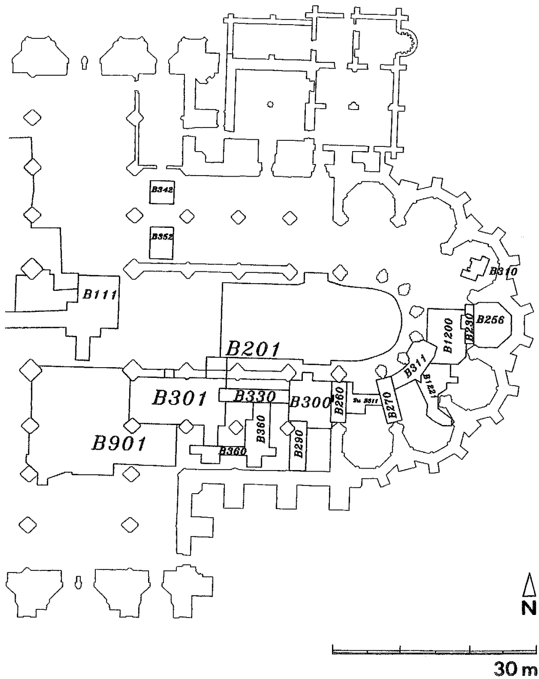
Taf. 5. Domgrabung Köln. Schematischer Grundriß der Ostteile mit den wichtigsten der als Befund bezeichneten Schnitten der Altgrabung (Ulrich Back). M. 1:500.
