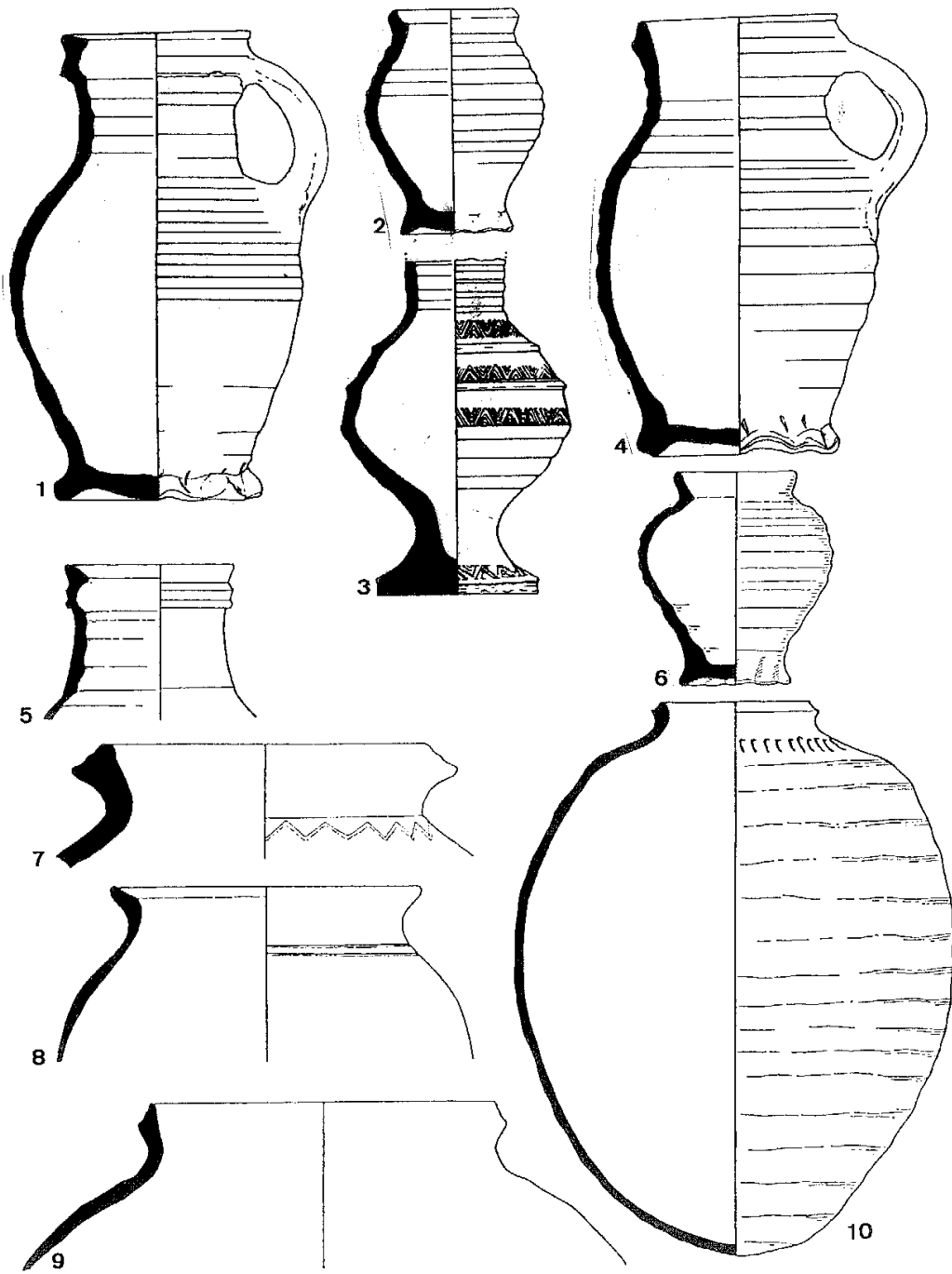
Taf. 39. 1-4 Junkersdorf (Stadt Köln), Keramik aus dem Grubenhaus am Statthalterhof (nach Steuer 1980, verändert). – 5-10 Lövenich (Stadt Köln), Keramik aus einem Grubenhaus (nach Bonner Jahrbücher 159, verändert). M. 1:3, 10 M. 1:6.
