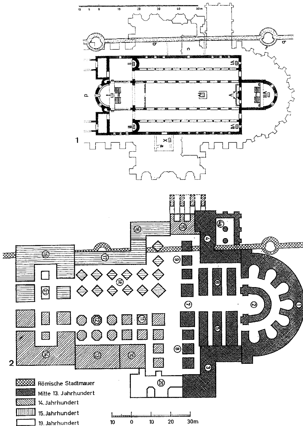
Taf. 46. 1 Köln, Alter Dom. Grundriß um 1245 (die Apsidiolen – vgl. B1240 – an den östlichen Querhausarmen sind noch nicht berücksichtigt). I bis X Altäre; a südlicher Portikus; b römische Stadtmauer; c Gerkammer (Sakristei); d Westatrium; e Kantharus (nach Weyres 1967a). M. 1:1000. – 2 Köln, gotischer Dom. Schematischer Fundamentplan (nach Wolff 1968). M. 1:1000.
