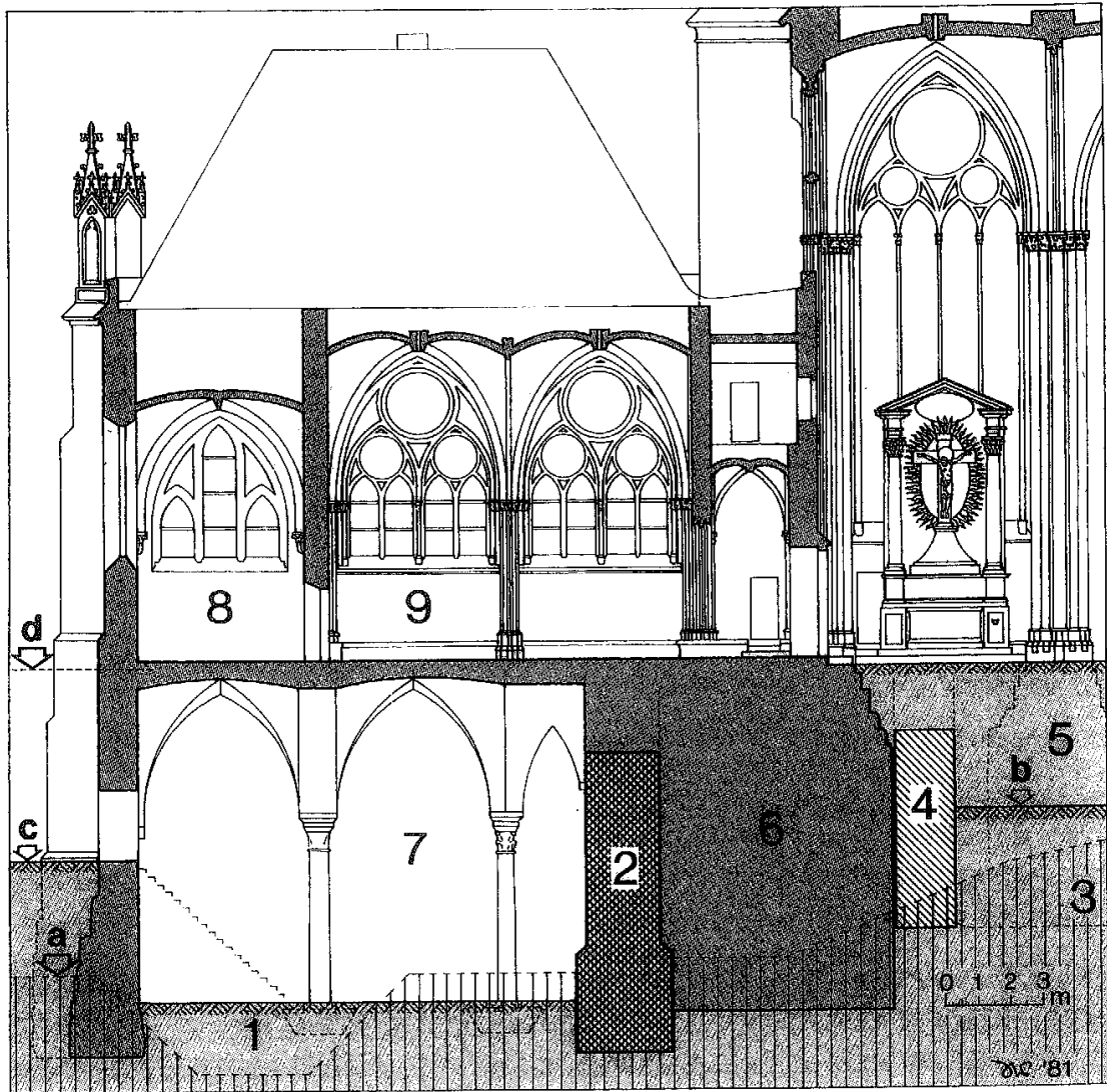
Taf. 48. Kölner Dom. N-S-Schnitt durch die Sakristei und das nördliche Joch des Querschiffes (vor 1868). 1 römischer Stadtmauergraben B1839; 2 römische Stadtmauer B1576; 3 vermutliches Geländeprofil vor dem Bau der römischen Stadtmauer (gewachsener Boden B1595); 4 Nordwand B1557 des Alten Domes; 5 Fundament B1545 des gotischen Pfeilers E 13; 6 Fundament B1553 der nördlichen Außenwand des gotischen Langchores; 7 Tiefkeller unter der Sakristei; 8 Sakristei-Nordbau (Archiv und Schatzkammer); 9 Sakristei (Kapitelsaal?); a Geländeoberkante in römischer Zeit; b Fußbodenniveau des Alten Domes B184/B1563); c Geländeoberkante vor 1868; d Geländeoberkante der Fußgängerzone an der Nordseite des Domes heute (nach Wolff 1989). M. 1:200.
