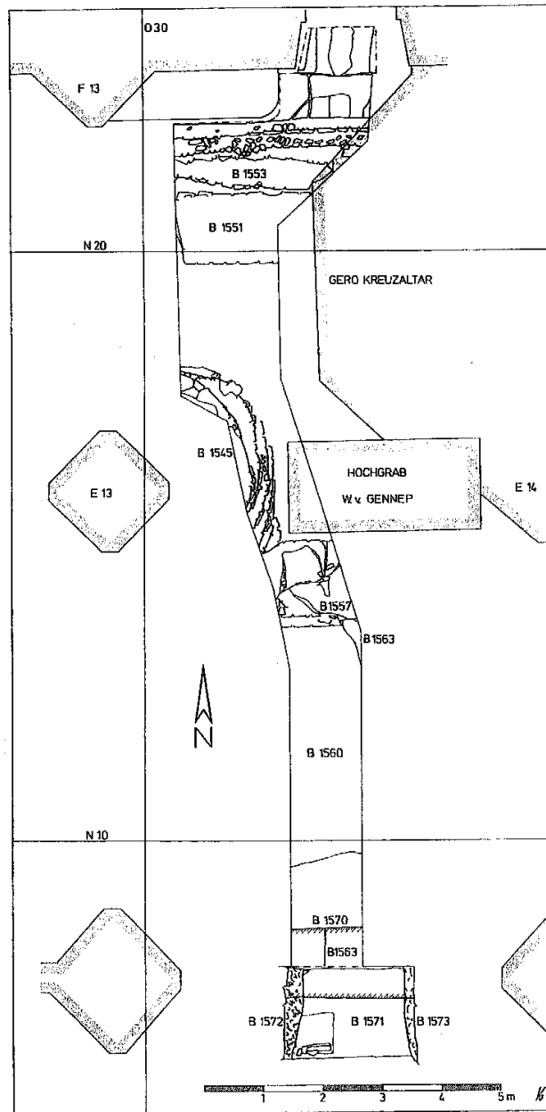
Taf. 56. Köln, Domgrabung. S-N-Stollen (sog. Kabelkanal) in den nördlichen Langchor-Seitenschiffen (Felder 53 und 54), Ausgrabung 1988 (nach Wolff 1988). M. 1:100.
