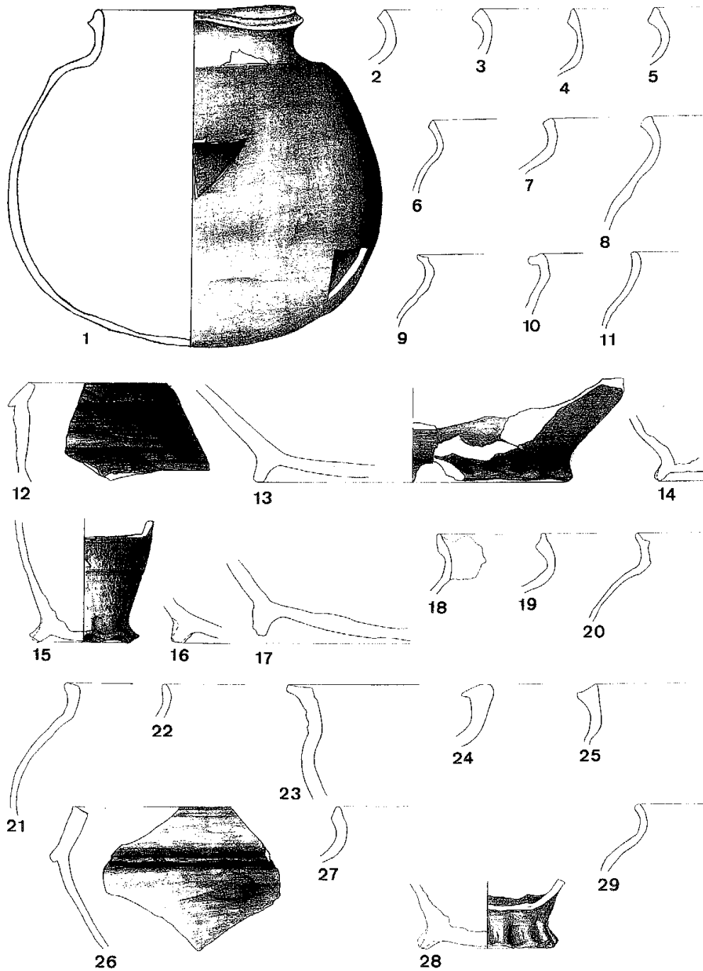
Taf. 9. Domgrabung Köln. Reduzierend gebrannte Irdenwaren (1-17 W 17; 18-22 W 18; 23-25 W 19; 26 W 20; 27 W 21; 28 W 22; 29 W 23). M. 1:3.
